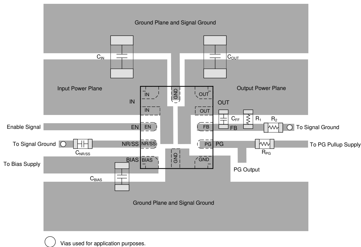
图 55. Example Layout
