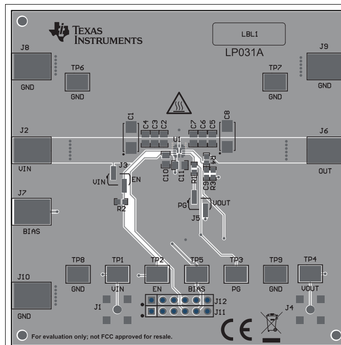
图 48. Top Composite View
