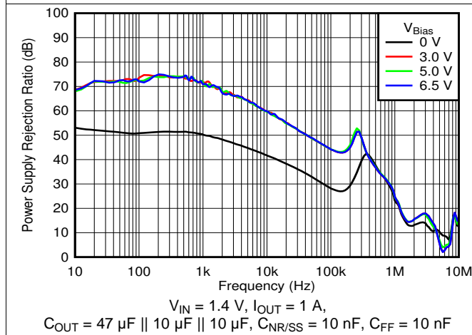
图 3. PSRR vs Frequency and V_{BIAS}
