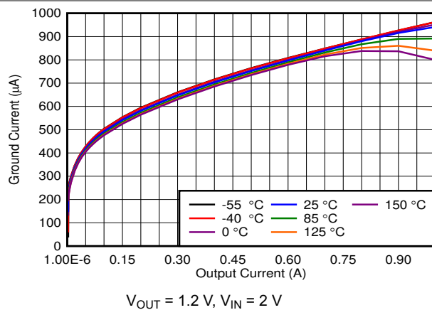
Figure 6-9. I_{\text{GND}} vs I_{\text{OUT}}
