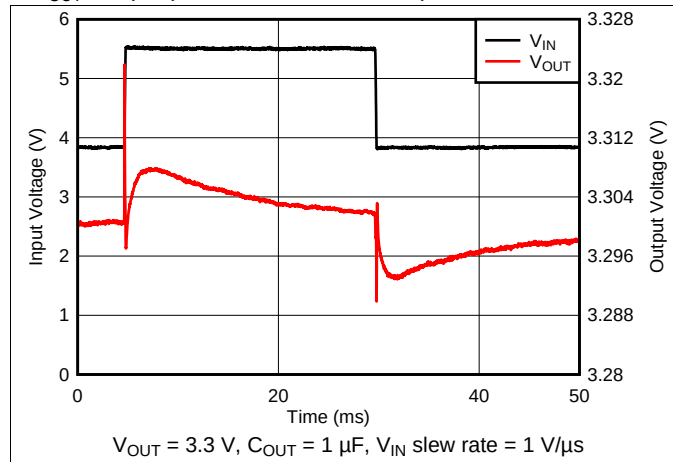
图 7. Line Transient
