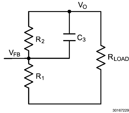
图 5: 设定 V_{OUT}
