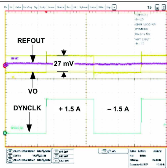
图 25. Transient Waveform
