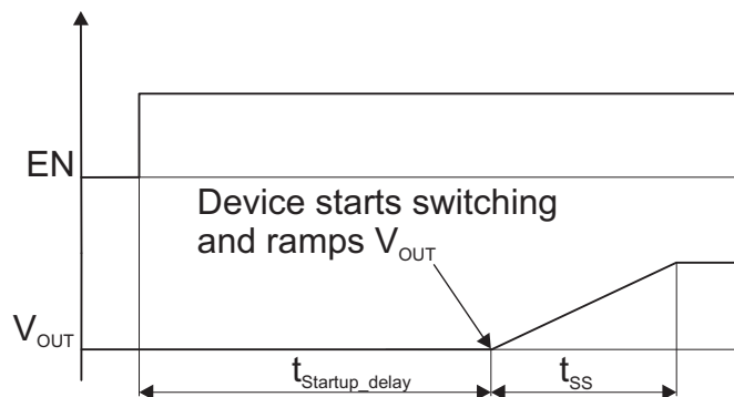
图 9. Device Startup
