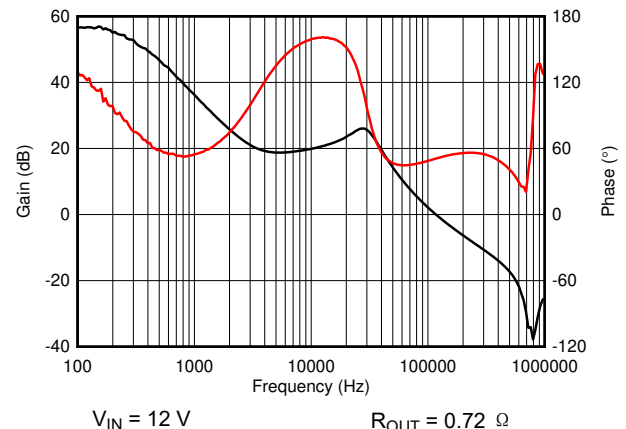
图 8-25. Bode Plot
