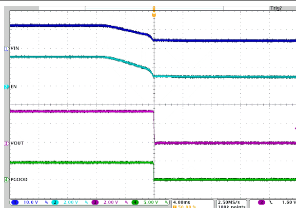
I_{OUT} = 1.5\text{ A} 图 8-13. VIN Shutdown
