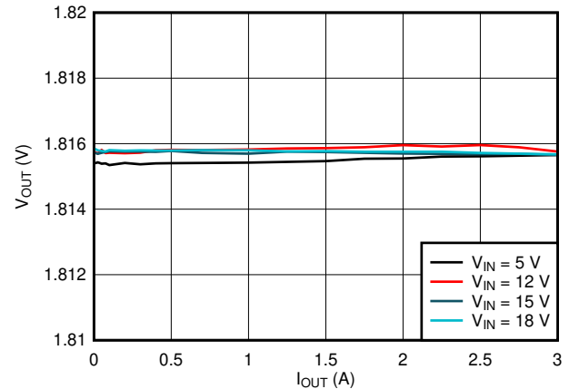
图 8-23. Load Regulation
