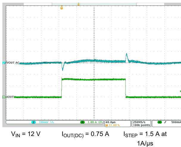
图 8-26. Load Transient
