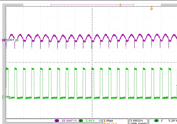
V_{IN} = 12\text{ V} I_{OUT} = 3\text{ A} 图 8-15. Output Ripple - 3-A Load
