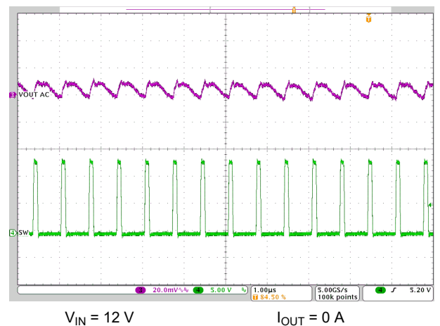
图 8-27. Output Ripple - No Load
