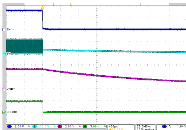
V_{IN} = 12\text{ V} I_{OUT} = 0\text{ A} 图 8-11. EN Shutdown
