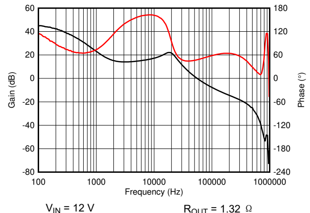
图 8-7. Bode Plot
