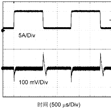
瞬态响应 V_{IN}=12V · V_{OUT}=1.2V 1至10A阶跃
