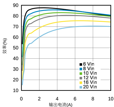
在85°C时2.5V输出效率
