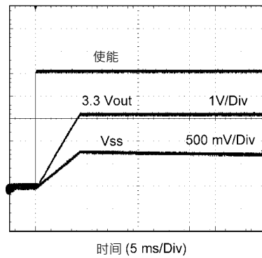
V_{OUT}=3.3 · 软启动, C_{SS} = 0.47\mu F
