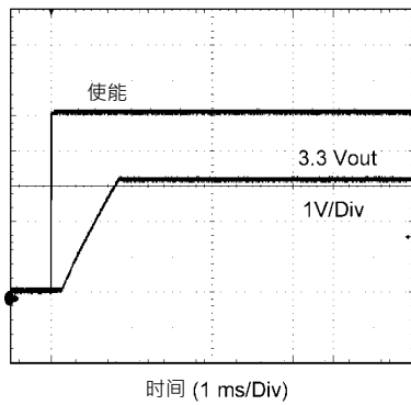
V_{OUT}=3.3 · 软启动,无CSS
