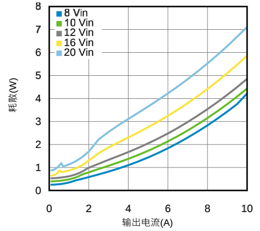
在25°C时5.0V输出耗散
