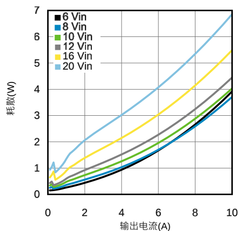
在25°C时1.8V输出耗散
