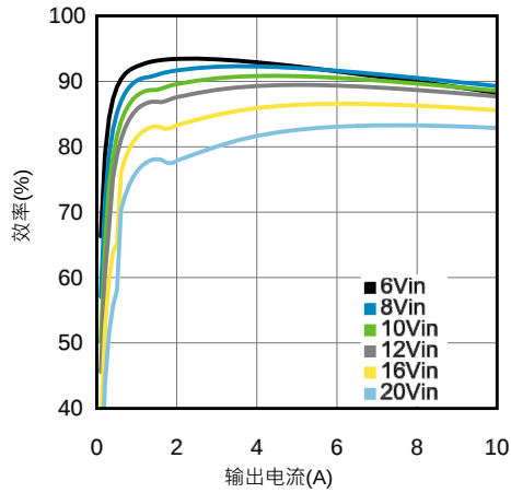
在25°C时3.3V输出效率
