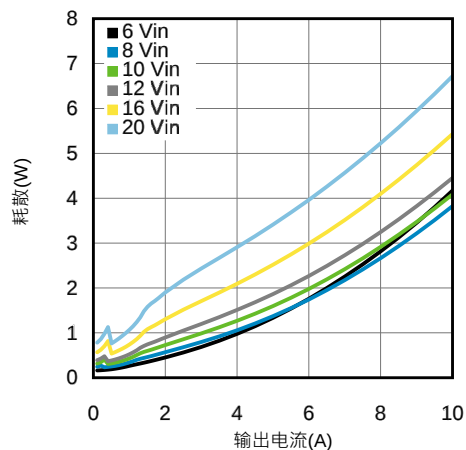
在25°C时2.5V输出耗散
