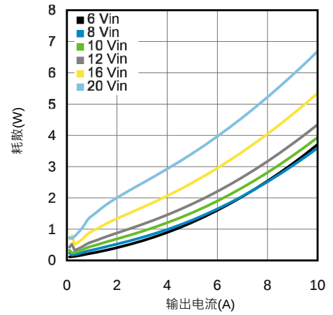
在25°C时1.2V输出耗散
