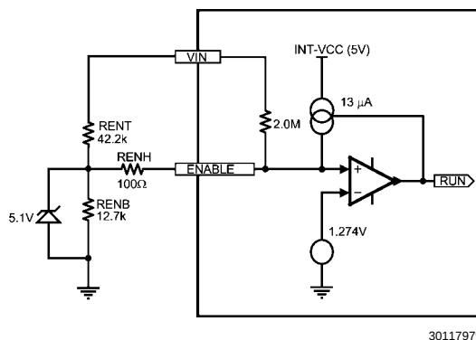
图1. 使能输入详图
