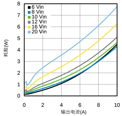
在85°C时1.5V输出耗散
