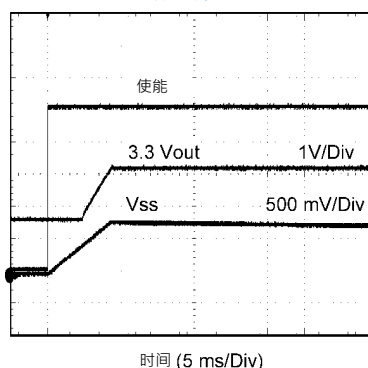
预偏置启动
