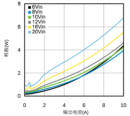
在25°C时3.3V输出耗散
