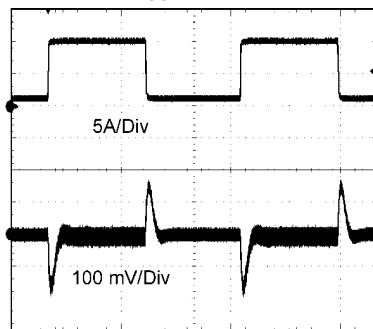
瞬态响应 V_{IN}=12V \cdot V_{OUT}=5.0V 1至10A阶跃
