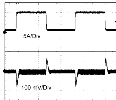
瞬态响应 V_{IN}=12V \cdot V_{OUT}=3.3V 1至10A阶跃
