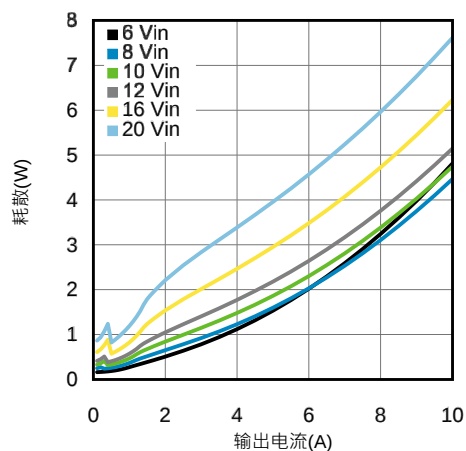
在85°C时2.5V输出耗散
