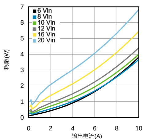
在25°C时1.5V输出耗散
