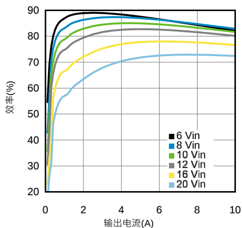
在25°C时1.8V输出效率
