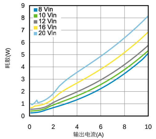
在85°C时5.0V输出耗散
