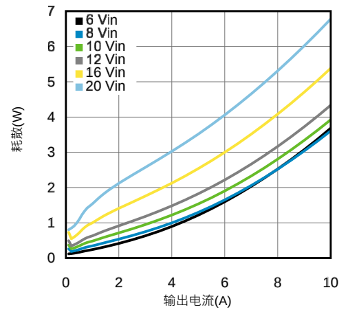
在25°C时1.0V输出耗散
