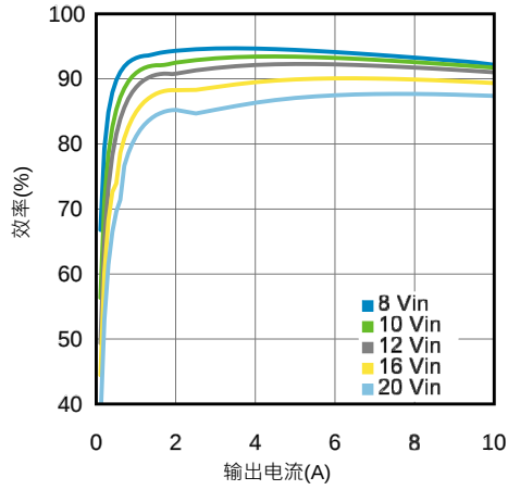
在25°C时5.0V输出效率
