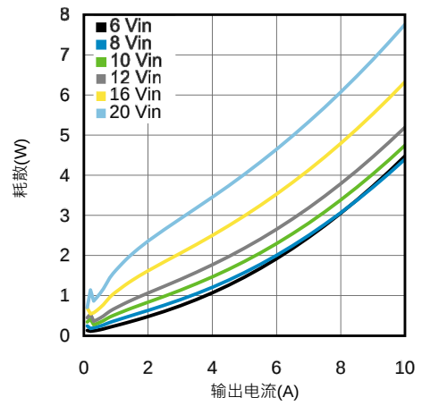
在85°C时1.2V输出耗散
