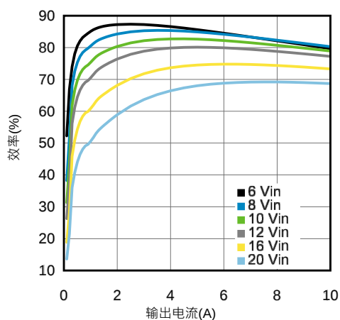
在25°C时1.5V输出效率
