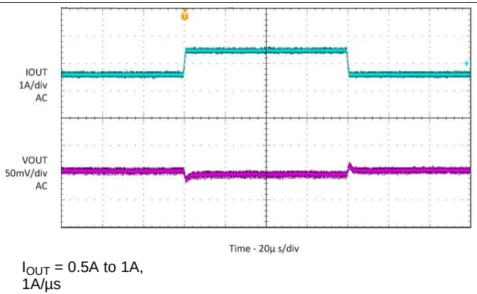
图 27. Load Transient
