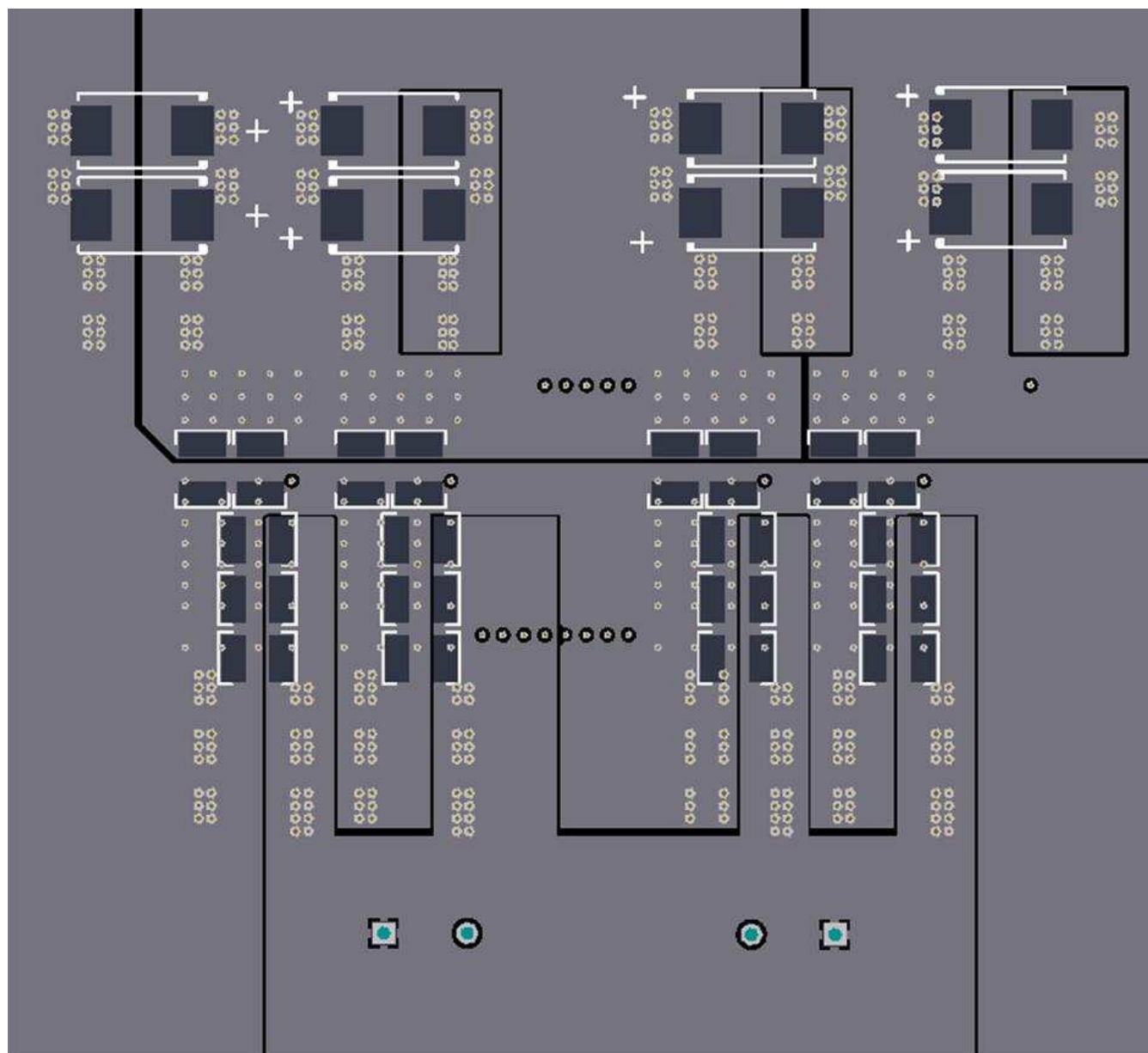
图 23. Bottom Layer (Top View)
