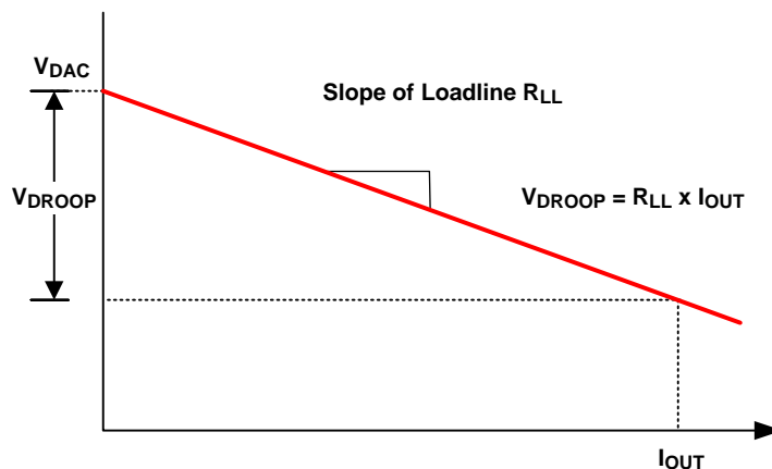
图 11. Load Line
