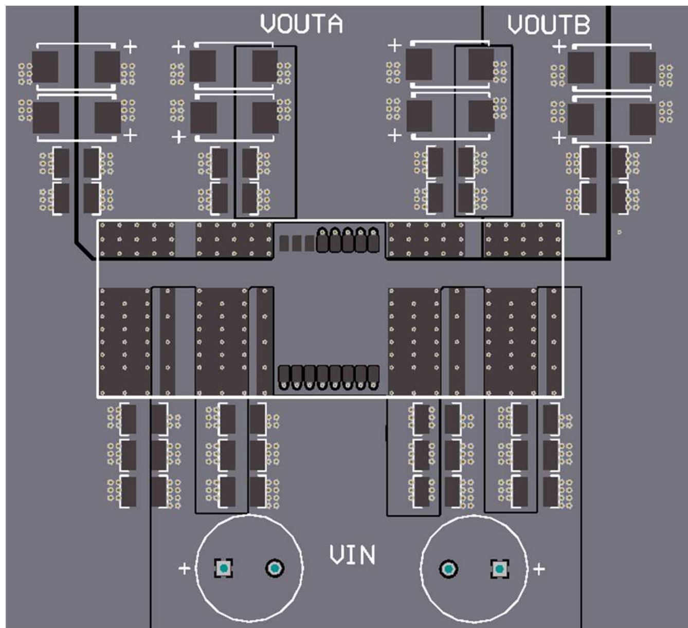
图 22. Top Layer (Top View)
