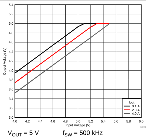
图 41. Voltage Dropout
