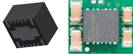
RLF 封装和典型布局
