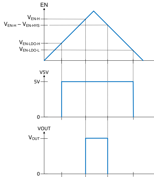
图 24. Precision Enable Behavior
