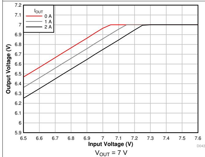
图 33. Voltage Dropout
