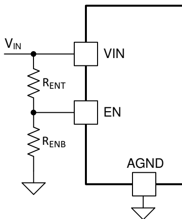
图 27. Adjustable UVLO
