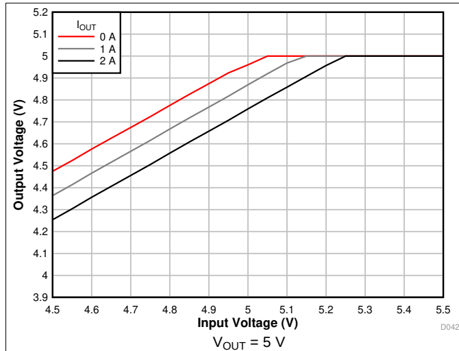
图 31. Voltage Dropout
