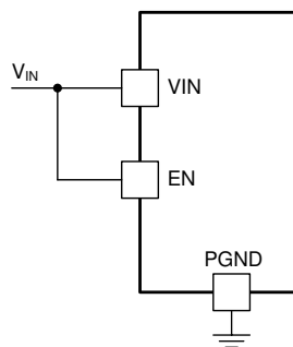
图 25. Enabling the Device
