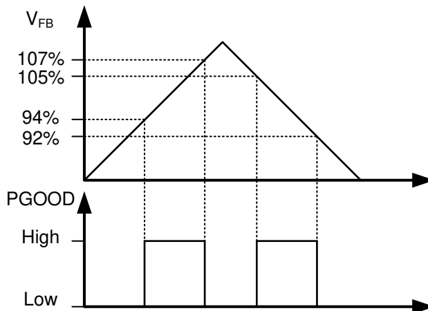
图 28. Power-good Flag
