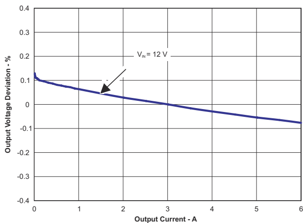
图 8-10. Load Regulation
