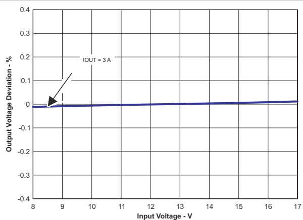
图 8-9. Line Regulation
