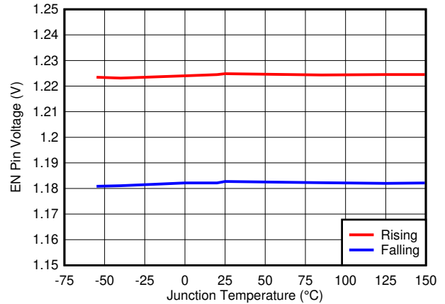
图 6-8. EN Pin UVLO Threshold vs Temperature
