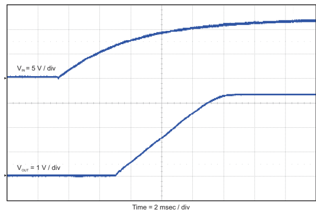
图 8-3. Start-Up With VIN
