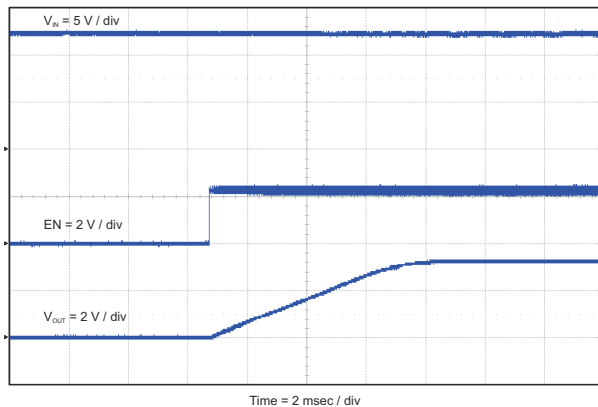
图 8-4. Start-Up With EN
