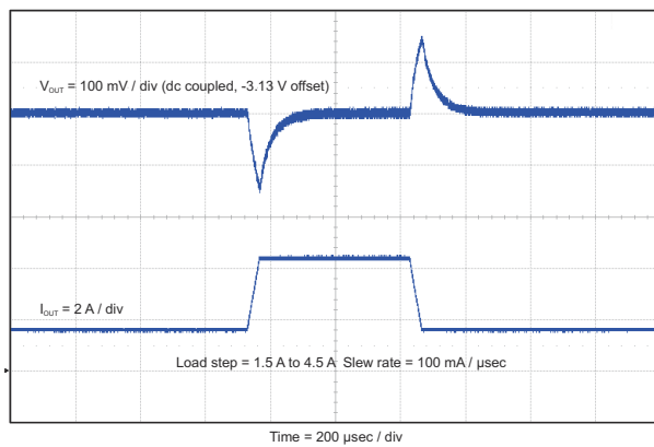
图 8-2. Load Transient
