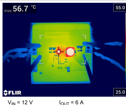
图 8-13. Thermal Image
