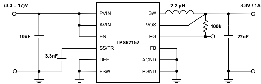
图 48. 3.3-V, 1-A Power Supply
