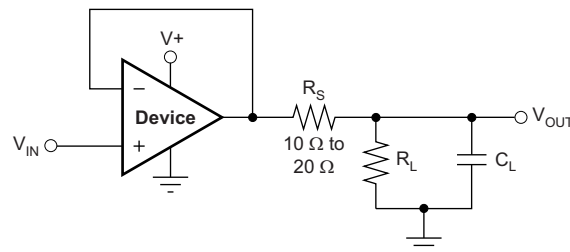
图 14. 改进电容负载驱动
