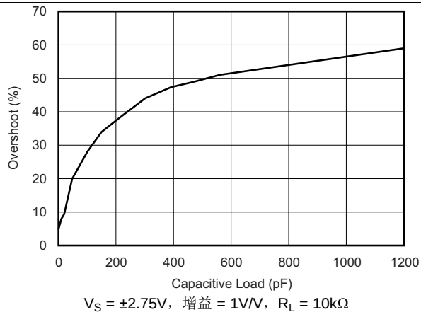
图 8. 小信号过冲与负载电容间的关系
