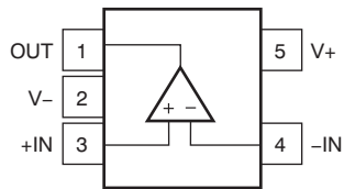
DBV 封装: TLV314
