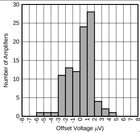
图 1. 偏移电压分布， V_S = 1.8\text{V}
