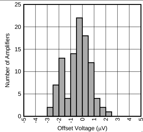
图 2. 偏移电压分布， V_S = 1.8\text{V}
