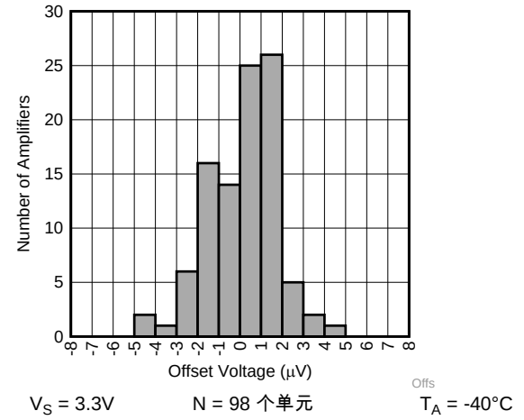
图 4. 偏移电压分布， V_S = 3.3\text{V}
