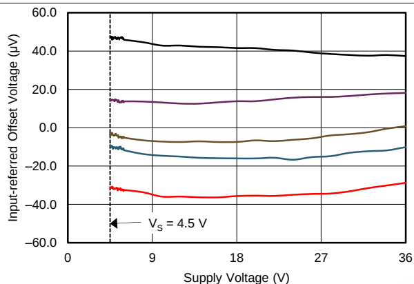
图 5. 失调电压与电源间的关系
