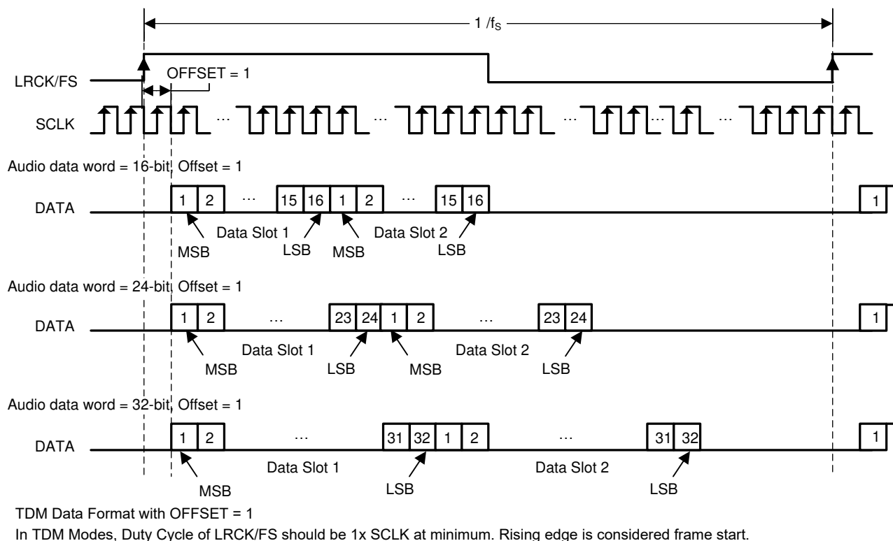
图 8-6. TDM 2 Audio Data Format
