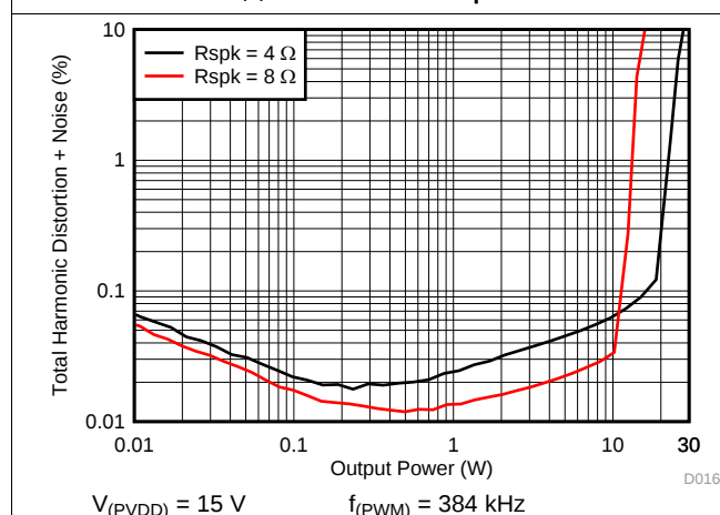
图 19. THD+N vs Output Power
