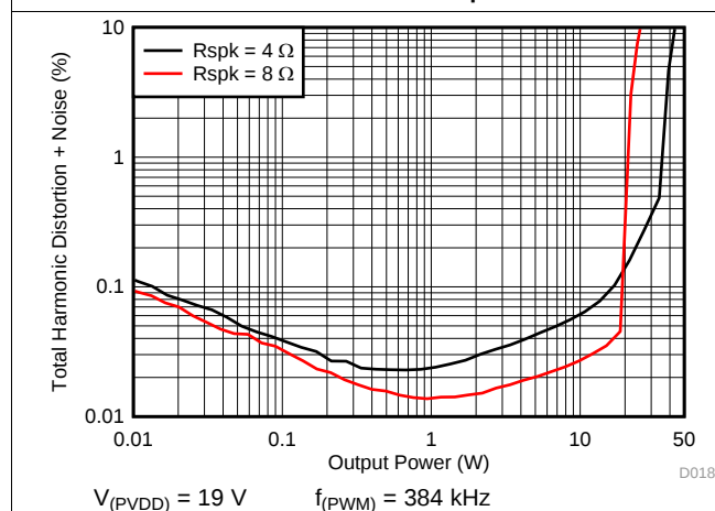
图 21. THD+N vs Output Power
