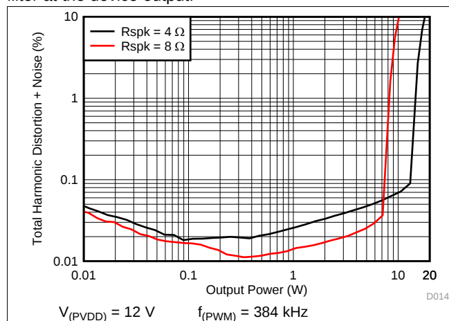
图 17. THD+N vs Output Power
