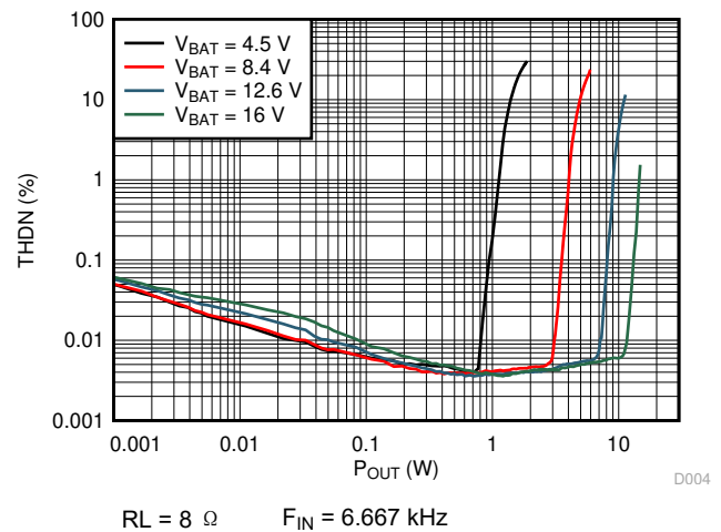
图 6-4. THD+N vs Output Power
