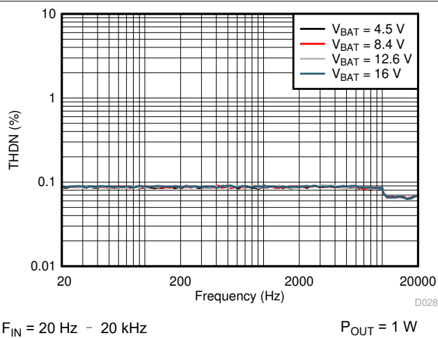
图 6-27. V_{SENSE} THD+N vs Frequency
