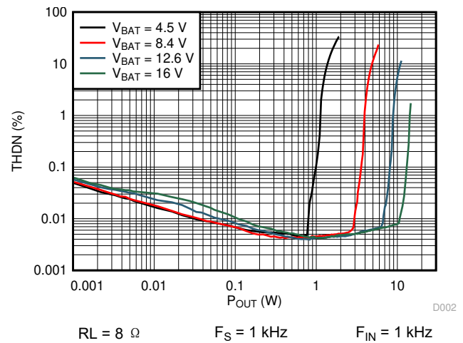
图 6-2. THD+N vs Output Power
