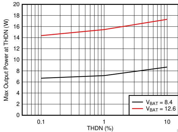
图 6-11. Max Output Power vs THD+N
