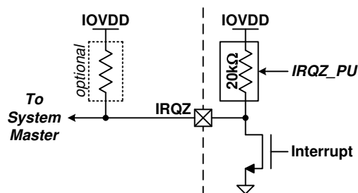
图 8-18. IRQZ Pin
