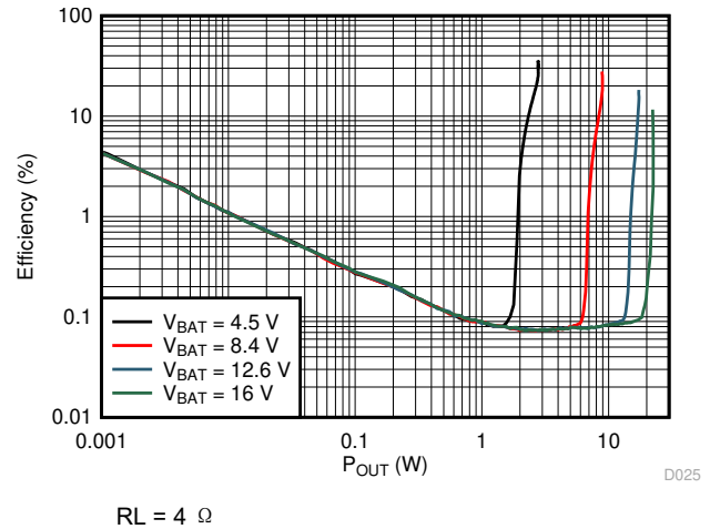
图 6-24. V_{SENSE} THD+N vs Output Power
