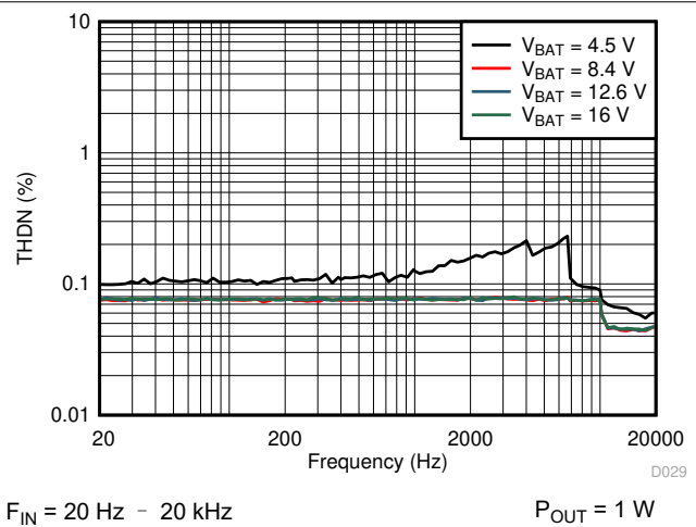
图 6-28. V_{SENSE} THD+N vs Frequency
