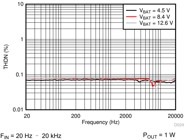
图 6-23. I_{SENSE} THD+N vs Frequency
