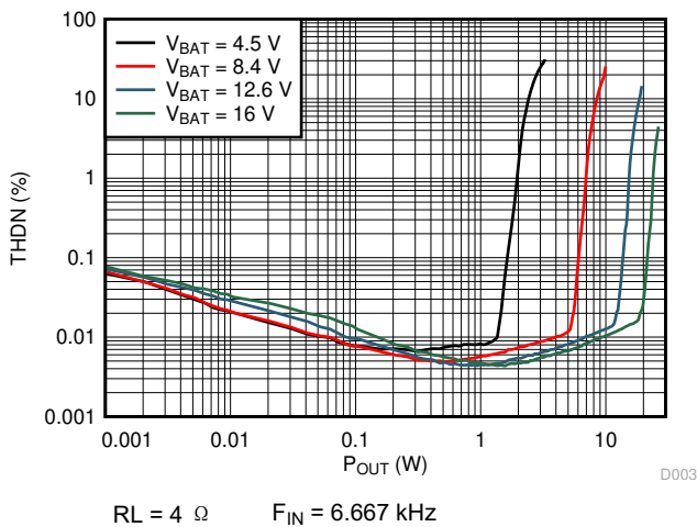
图 6-3. THD+N vs Output Power
