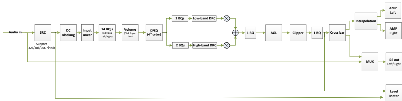
图 7-7. Audio Process Flow
