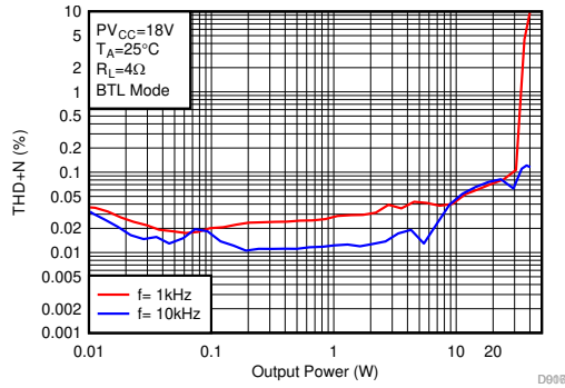
图 6-9. THD+N vs Output Power-BTL
