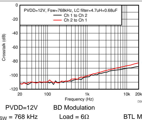
图 64. Crosstalk
