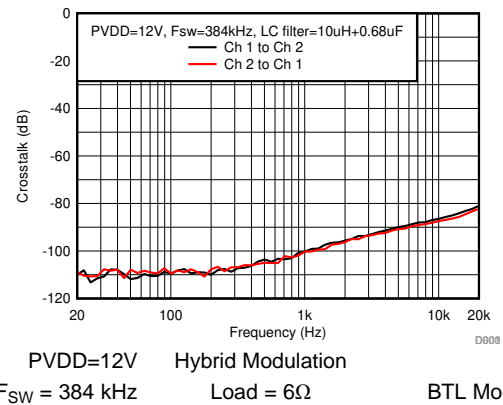
图 18. Crosstalk
