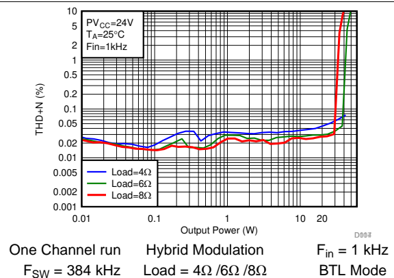
图 16. THD+N vs Output Power-BTL
