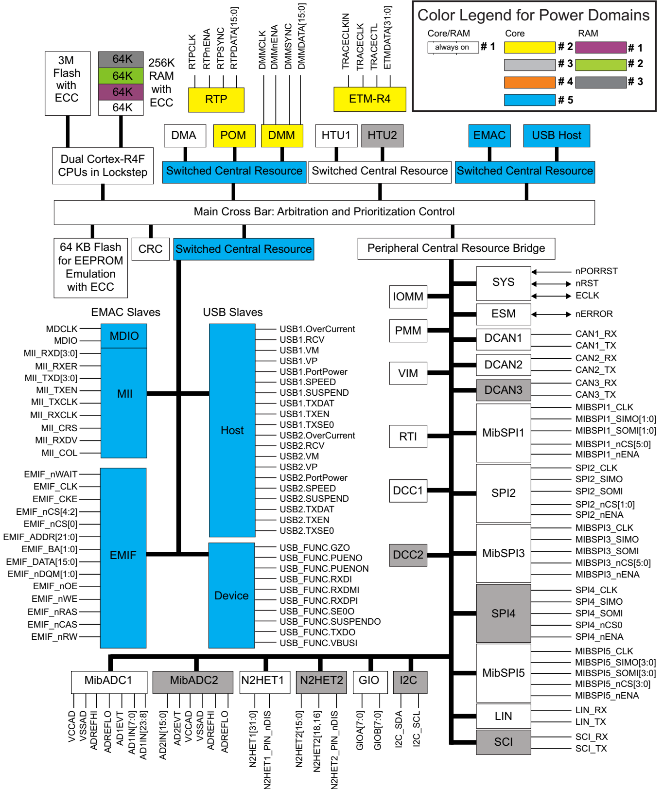
图 1-1. 功能方框图
