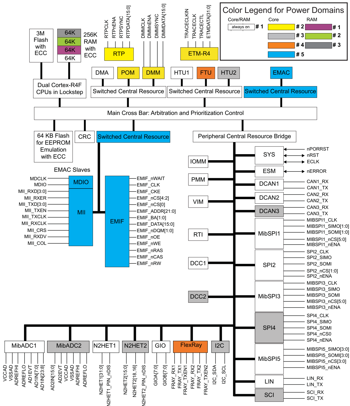
图 1-1. 功能方框图
