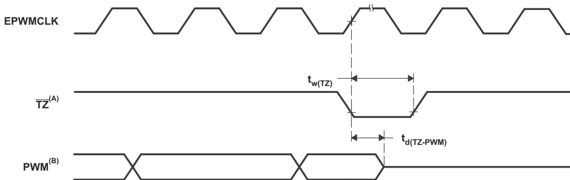
图 7-53. PWM Hi-Z Characteristics
