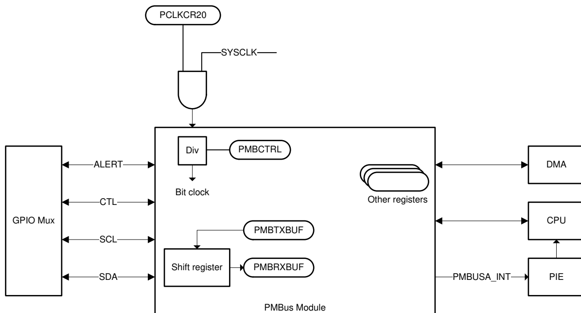
图 7-75. PMBus Block Diagram
