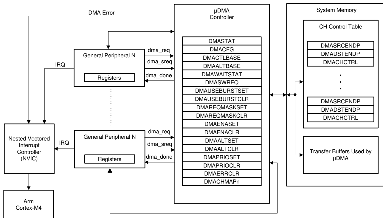
图 8-14. μDMA Block Diagram
