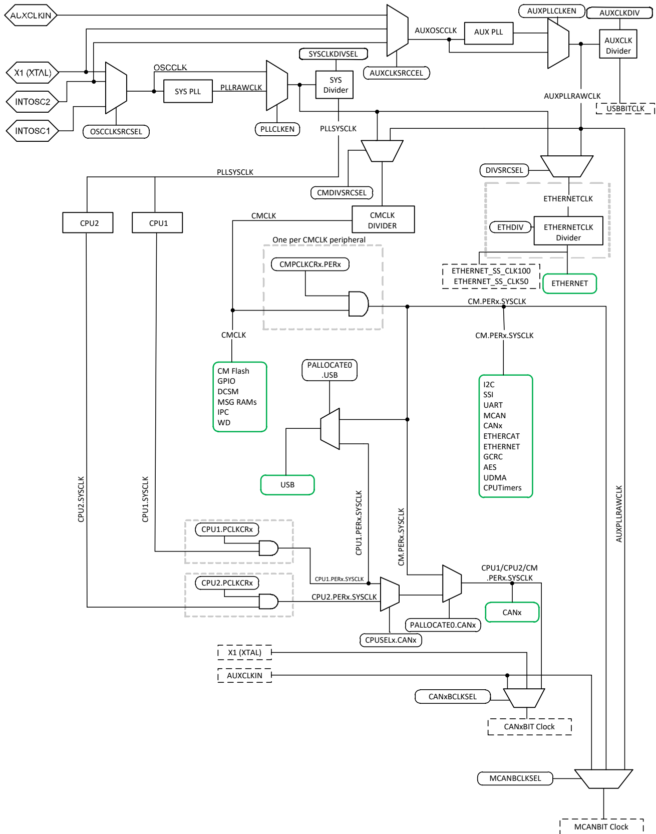
图 8-15. Clocking System
