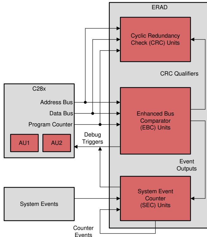
图 8-2. ERAD Overview
