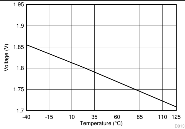
图 15. V_{OL,off}
