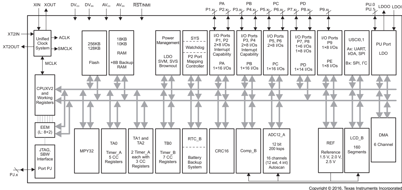
图 1-2. 功能框图 – MSP430F6435 和 MSP430F6433
