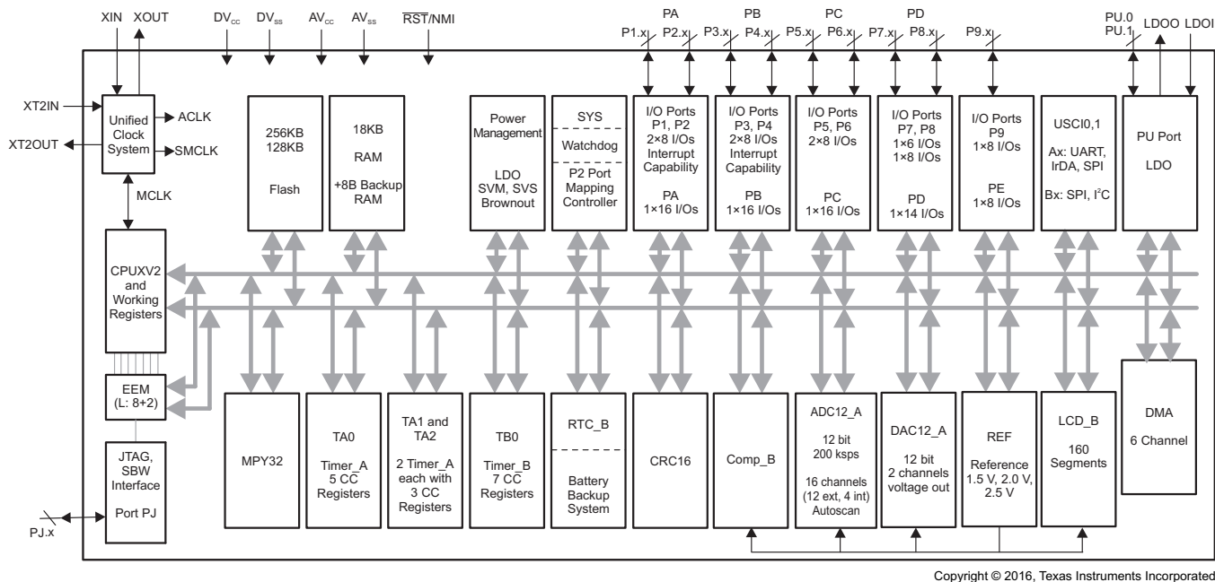
图 1-1. 功能框图 – MSP430F6438 和 MSP430F6436
