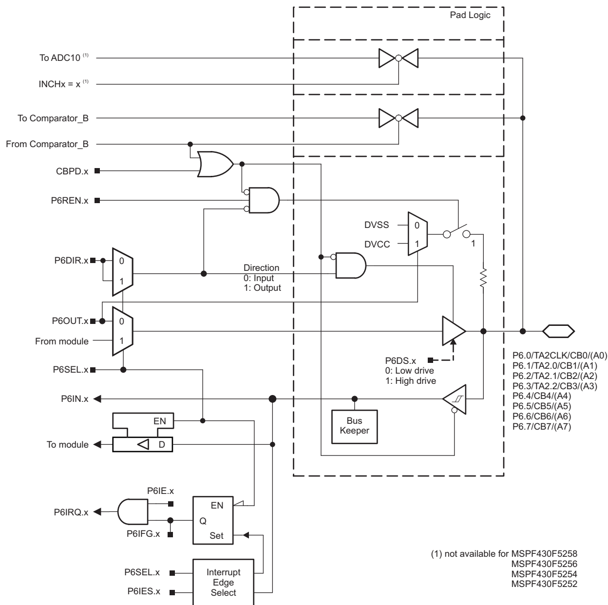
图 6-11. Port P6 (P6.0 to P6.7) Diagram
