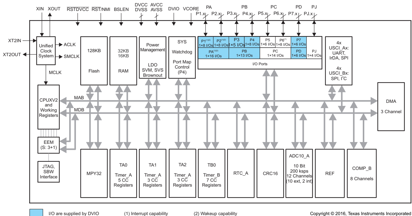
图 1-1. 功能方框图
