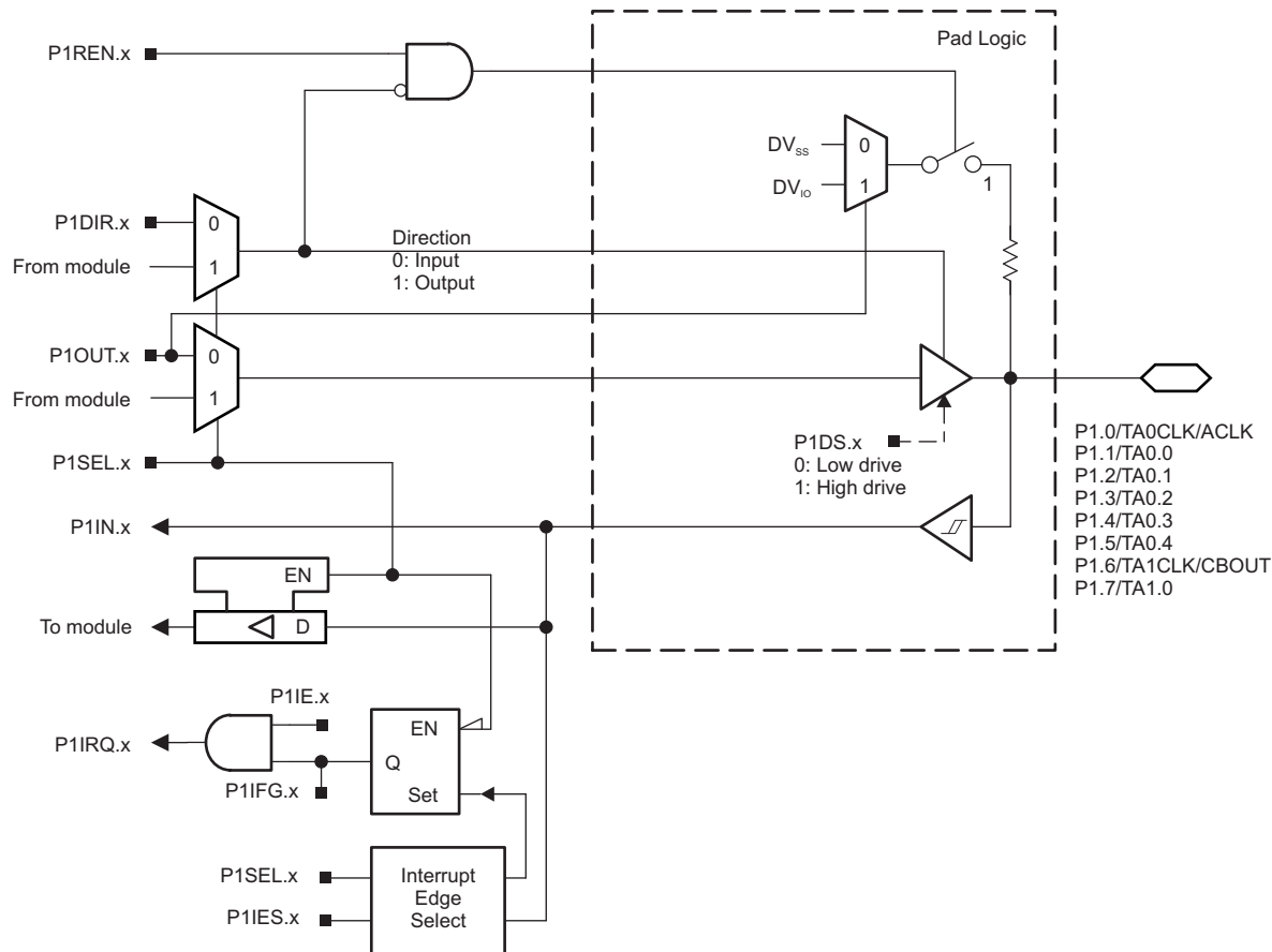
图 6-2. Port P1 (P1.0 to P1.7) Diagram
