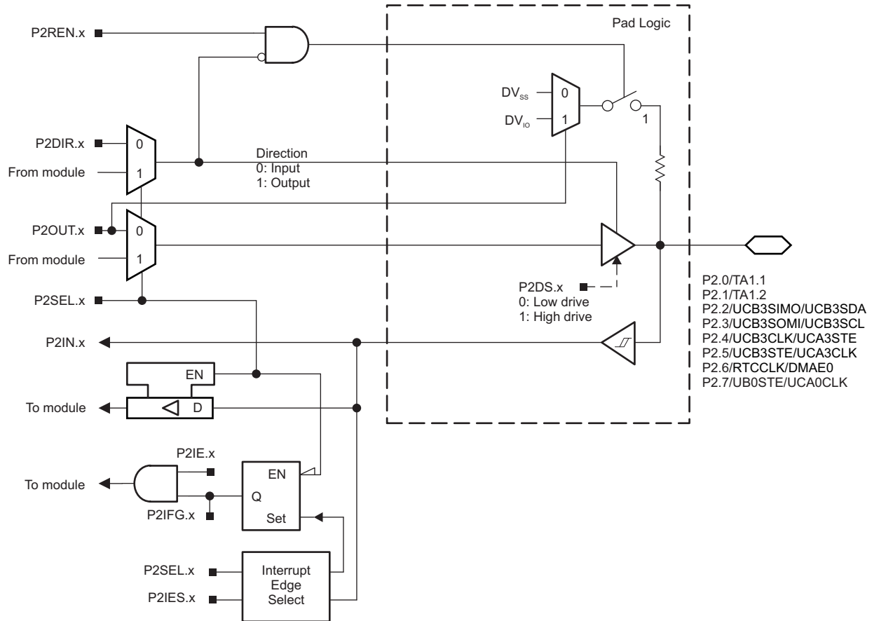
图 6-3. Port P2 (P2.0 to P2.7) Diagram
