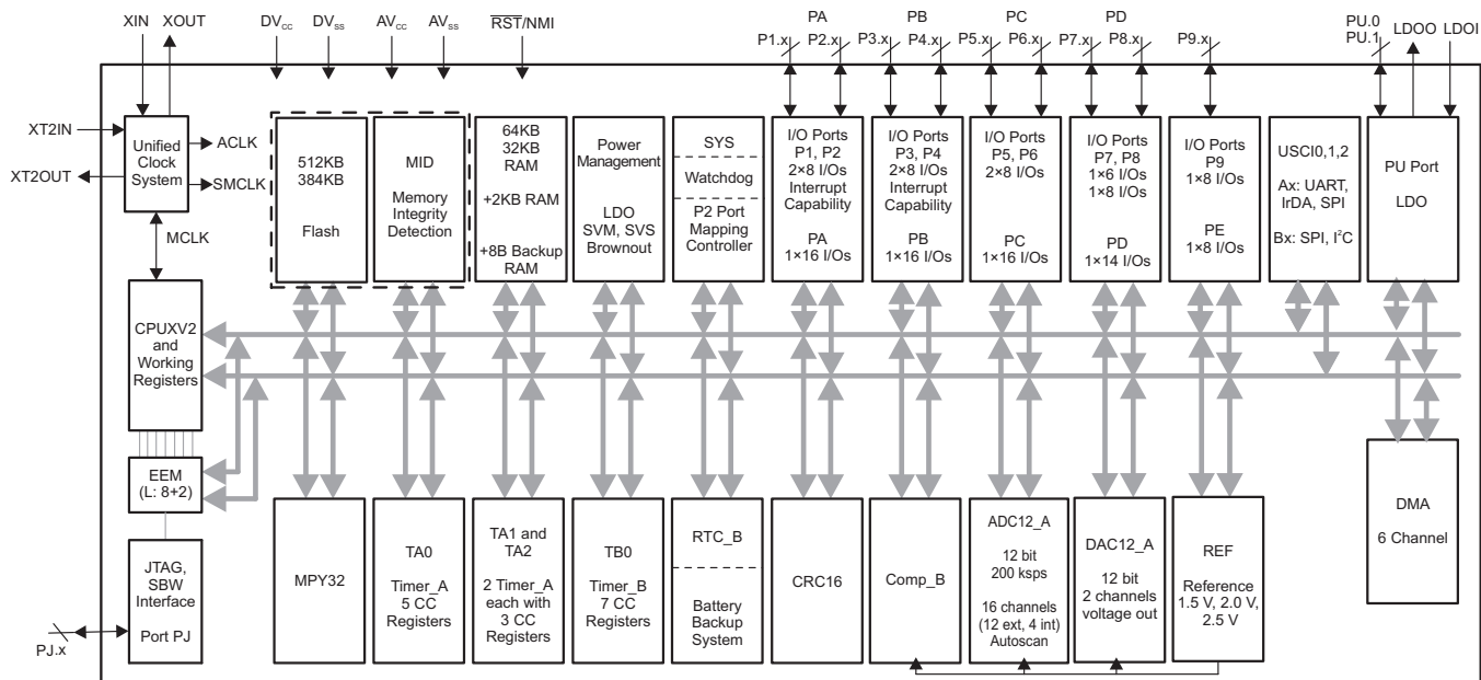
图 1-4. 功能方框图 – MSP430F5359、MSP430F5358
