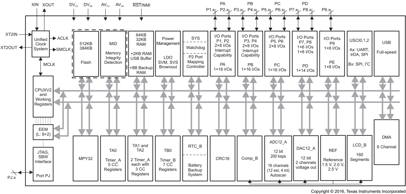
图 1-1. 功能方框图 – MSP430F6659、MSP430F6658
