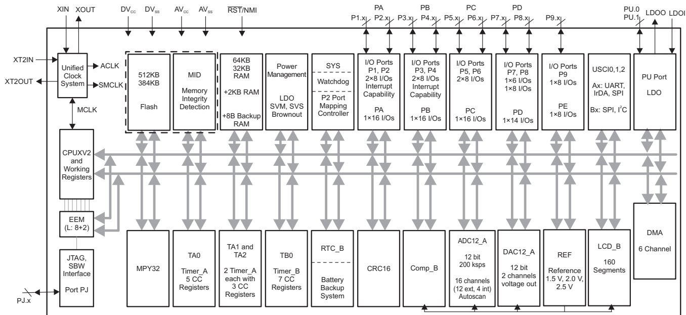
图 1-2. 功能方框图 – MSP430F6459、MSP430F6458
