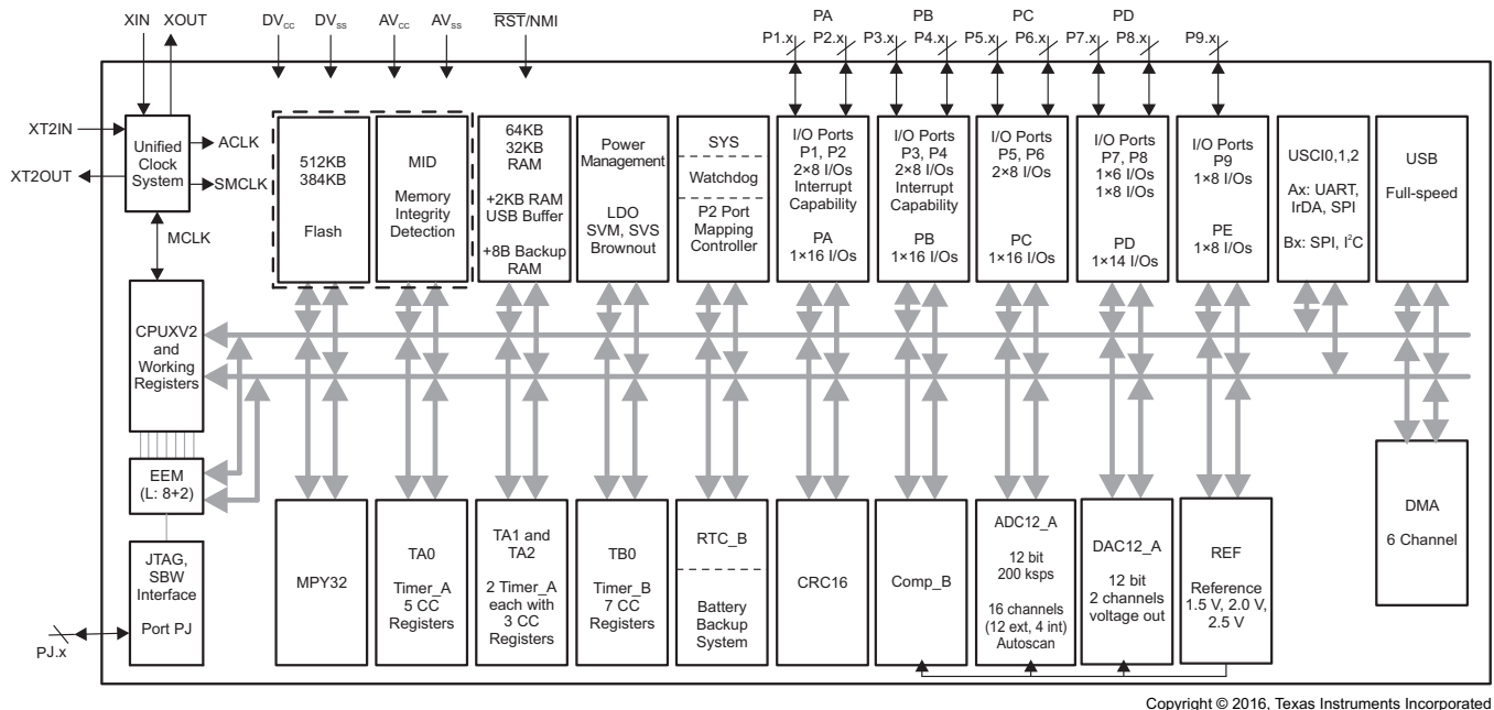
图 1-3. 功能方框图 – MSP430F5659、MSP430F5658
