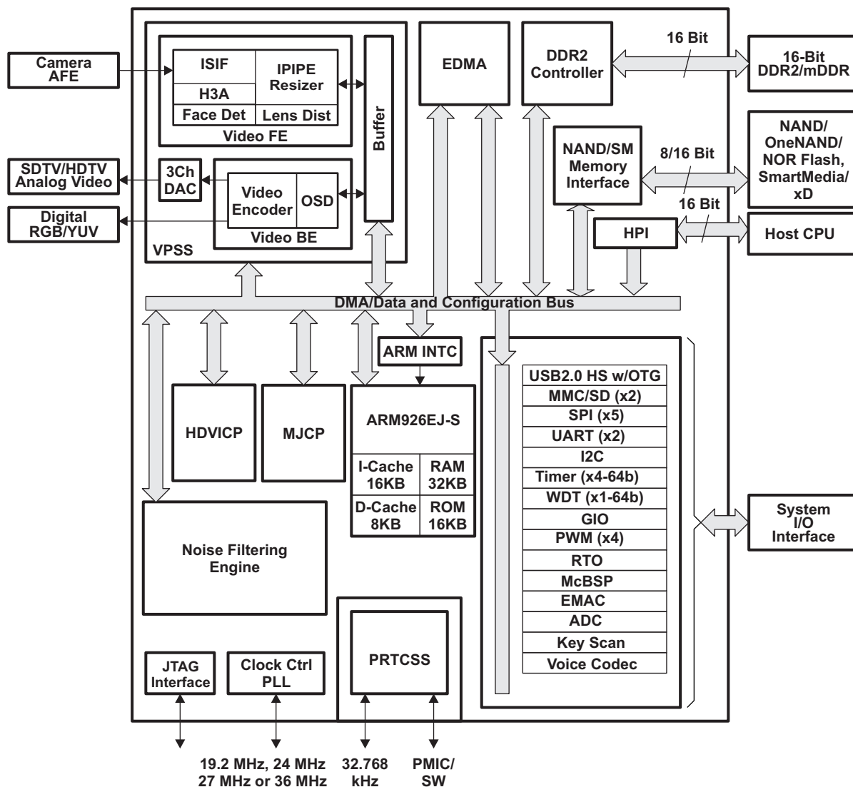
图 1-1. 功能方框图
