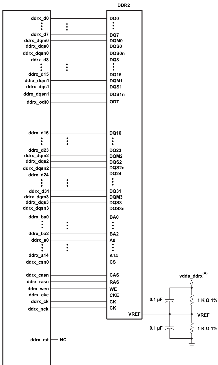
PCB_DDR2_1
