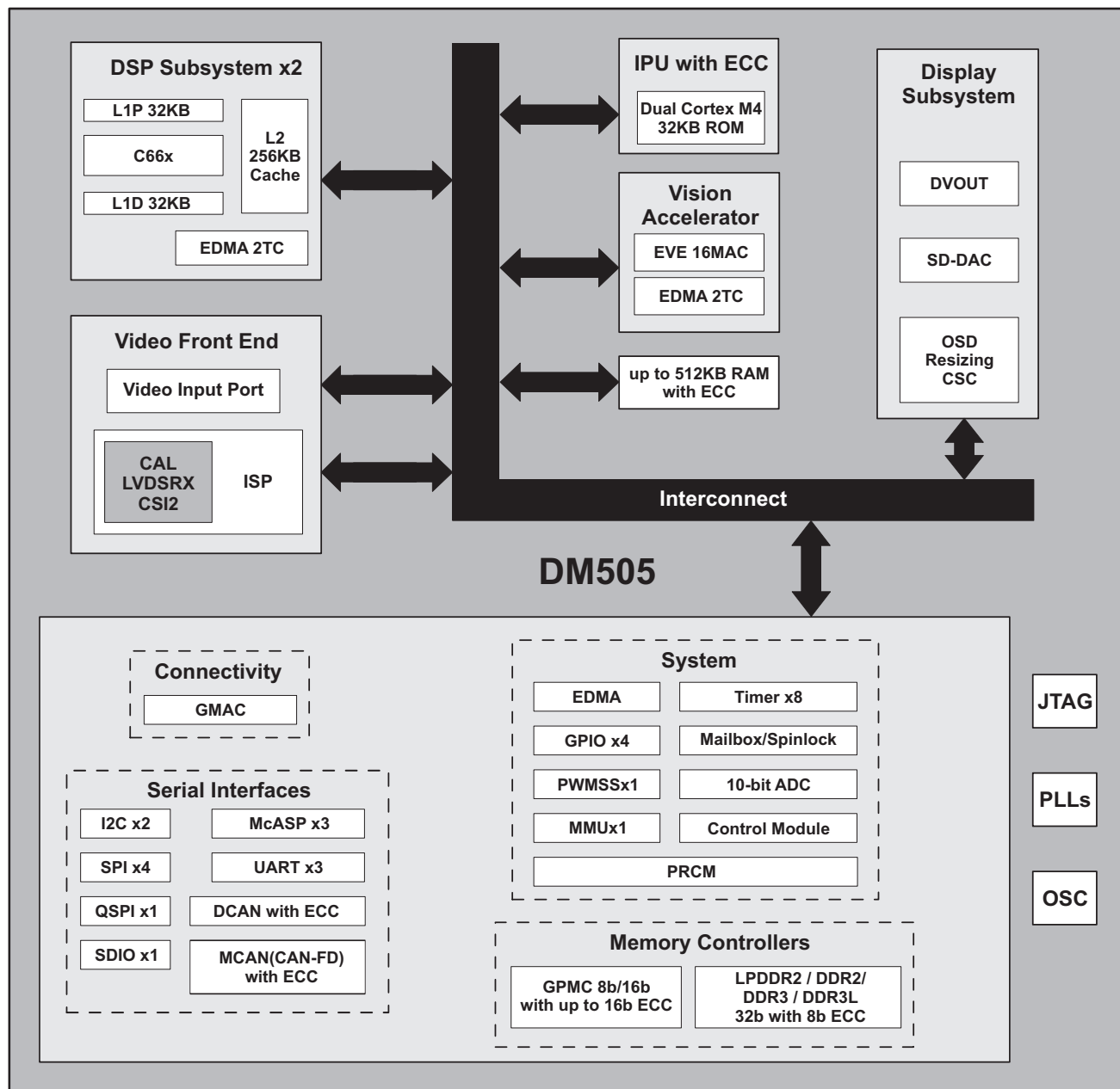
图 1-1. DM505 方框图
