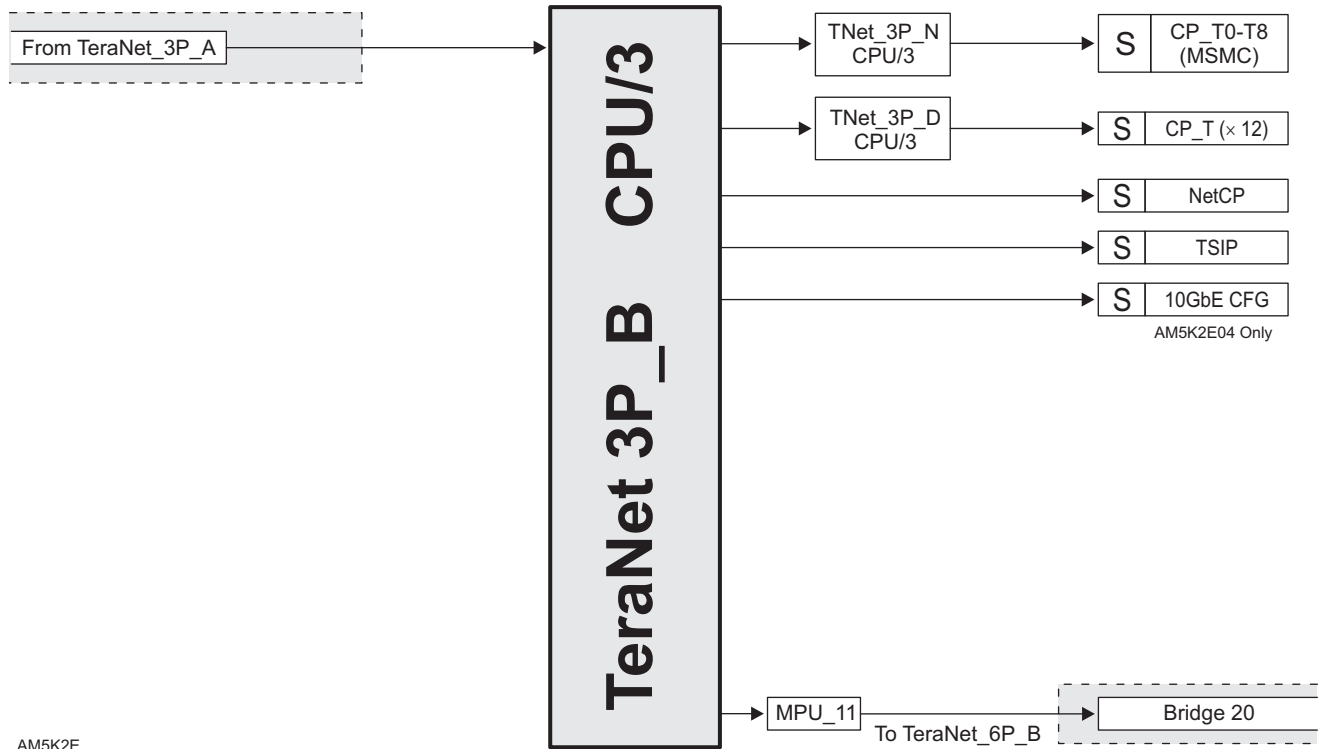
图 7-5. TeraNet 3P_B
