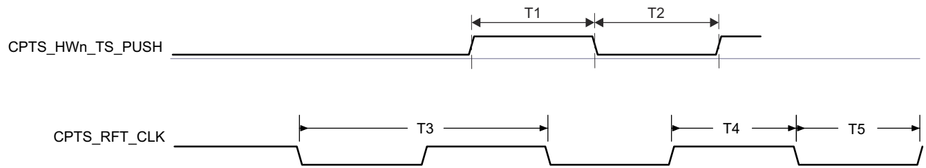
图 8-93. CPTS Input Timing
