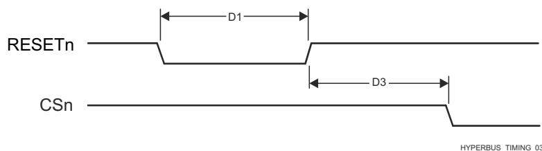
图 8-64. HyperBus Timing Diagrams – Reset
