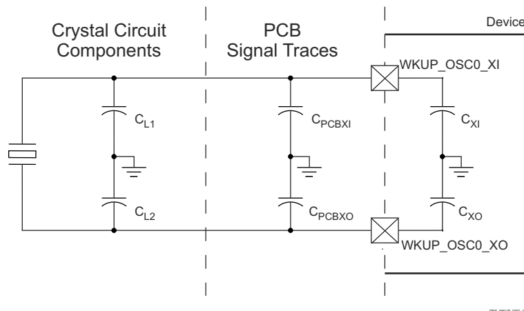
图 8-16. Load Capacitance
