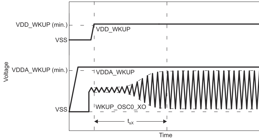
图 8-15. WKUP_OSC0 Start-up Time
