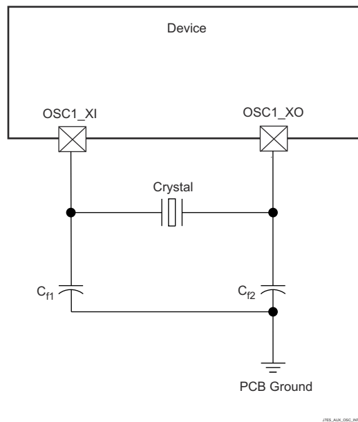
图 8-19. OSC1 Crystal Implementation
