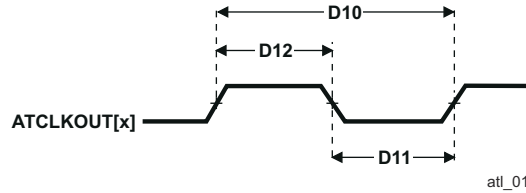
图 8-28. ATCLKOUT[x] Timing
