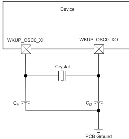
图 8-14. WKUP_OSC0 Crystal Implementation
