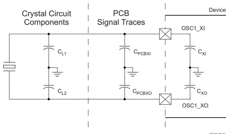
图 8-21. Load Capacitance
