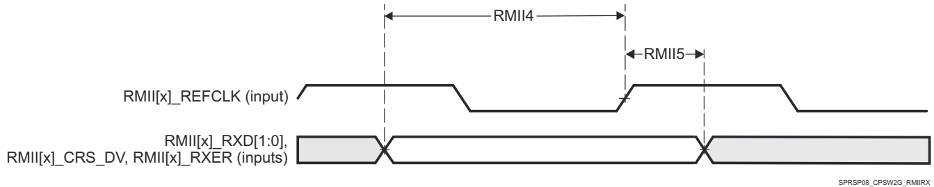
图 8-36. RMII[x]_RXD[1:0], RMII[x]_CRS_DV, RMII[x]_RXER Timing - RMII Mode
