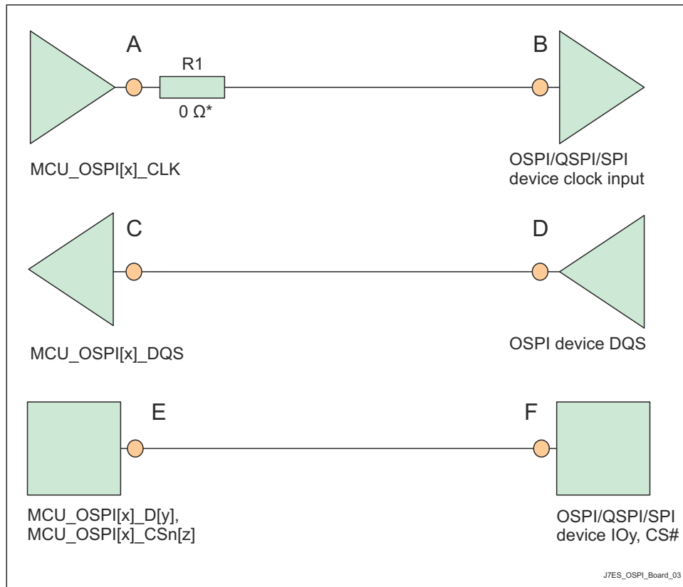
图 10-4. OSPI Interface High Level Schematic
