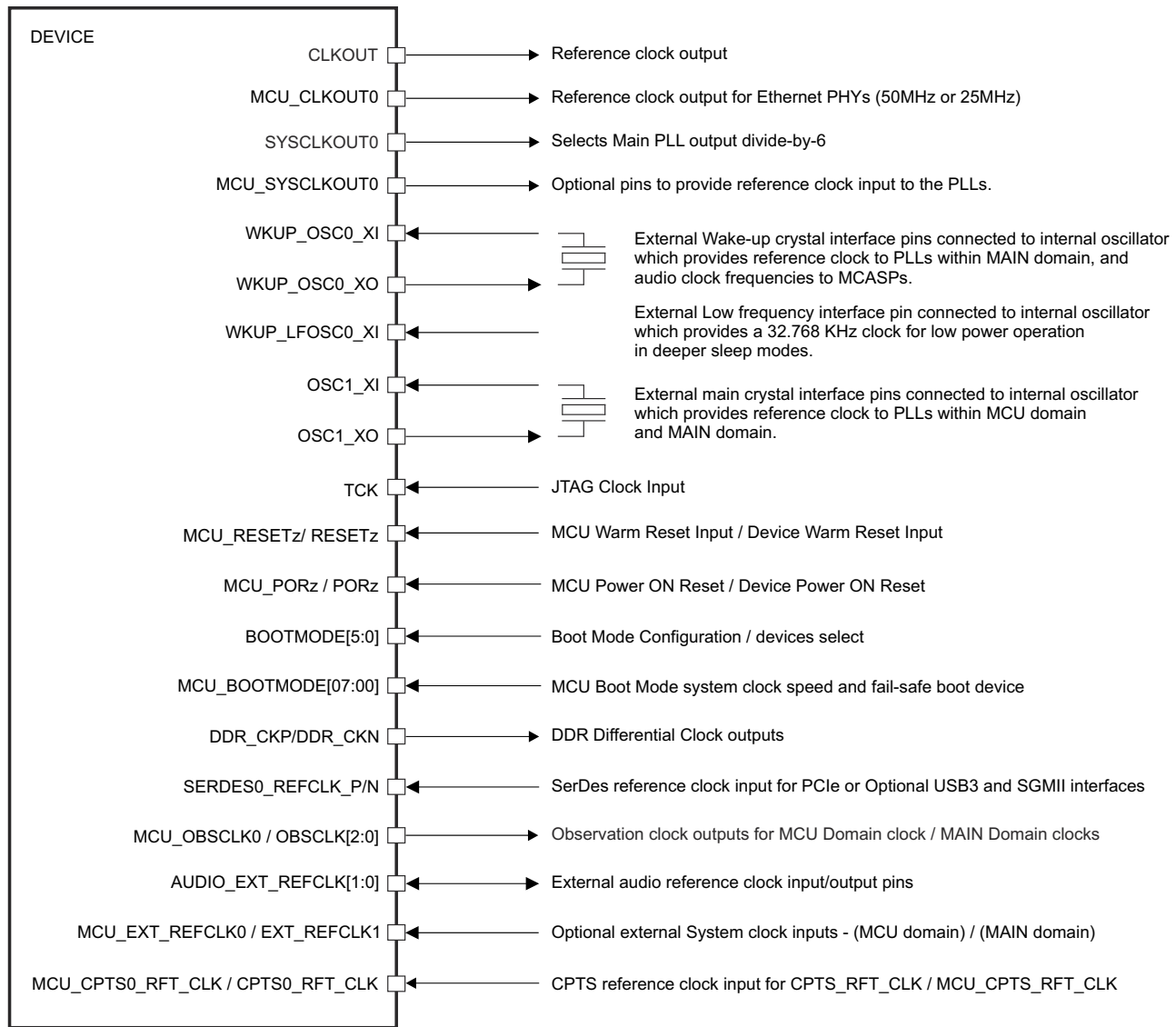
图 8-13. Input Clocks Interface
