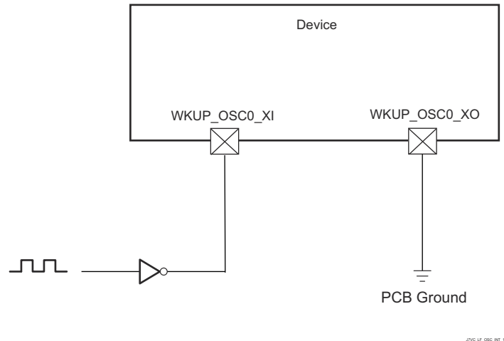
图 8-18. 1.8-V LVC MOS-Compatible Clock Input
