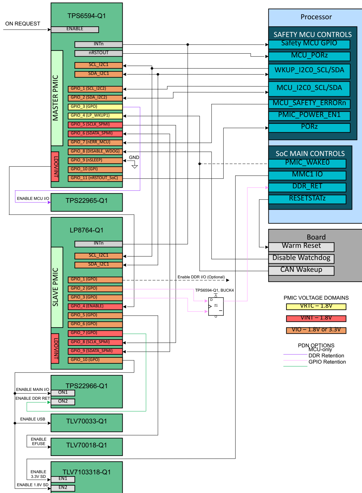
图 10-1. TPS6594-Q1 and LP8764-Q1 Digital Connections
