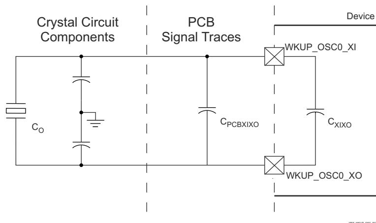
图 8-17. Shunt Capacitance
