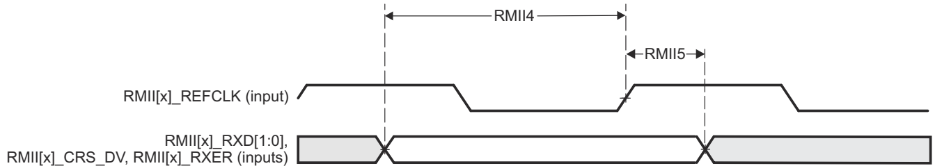
图 8-30. RMII[x]_RXD[1:0], RMII[x]_CRS_DV, RMII[x]_RXER Timing – RMII Mode
