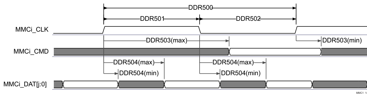
图 8-92. SD/SDIO - High Speed SD - DDR - Data/Command Transmit
