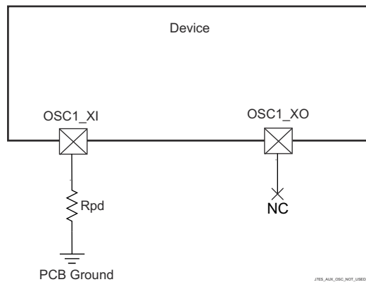
图 8-24. OSC1 Not Used
