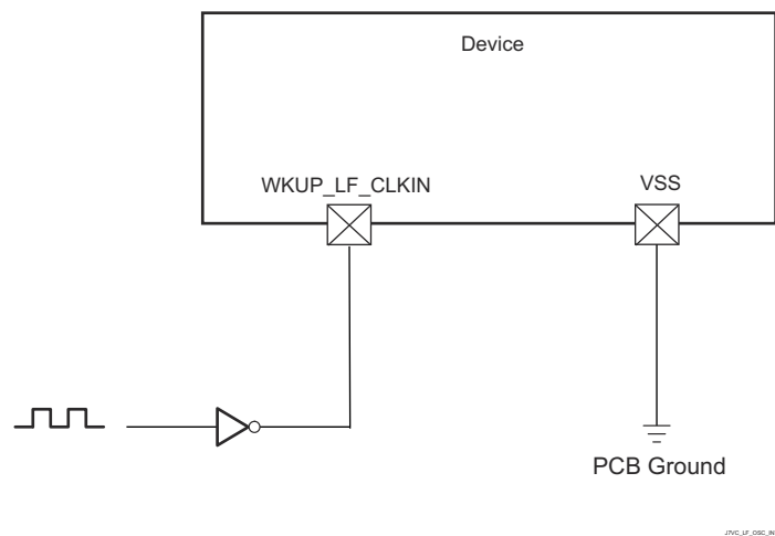
图 8-25. WKUP_LF_CLKIN Crystal Implementation
