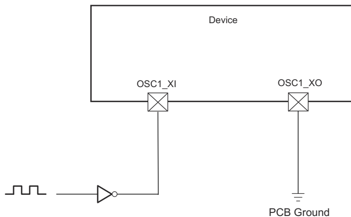
图 8-23. 1.8-V LVCMOS-Compatible Clock Input
