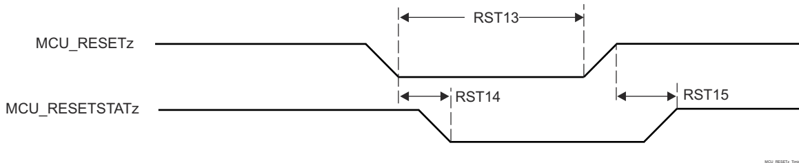
图 8-11. MCU_RESETz and MCU_RESETSTATz Timing
