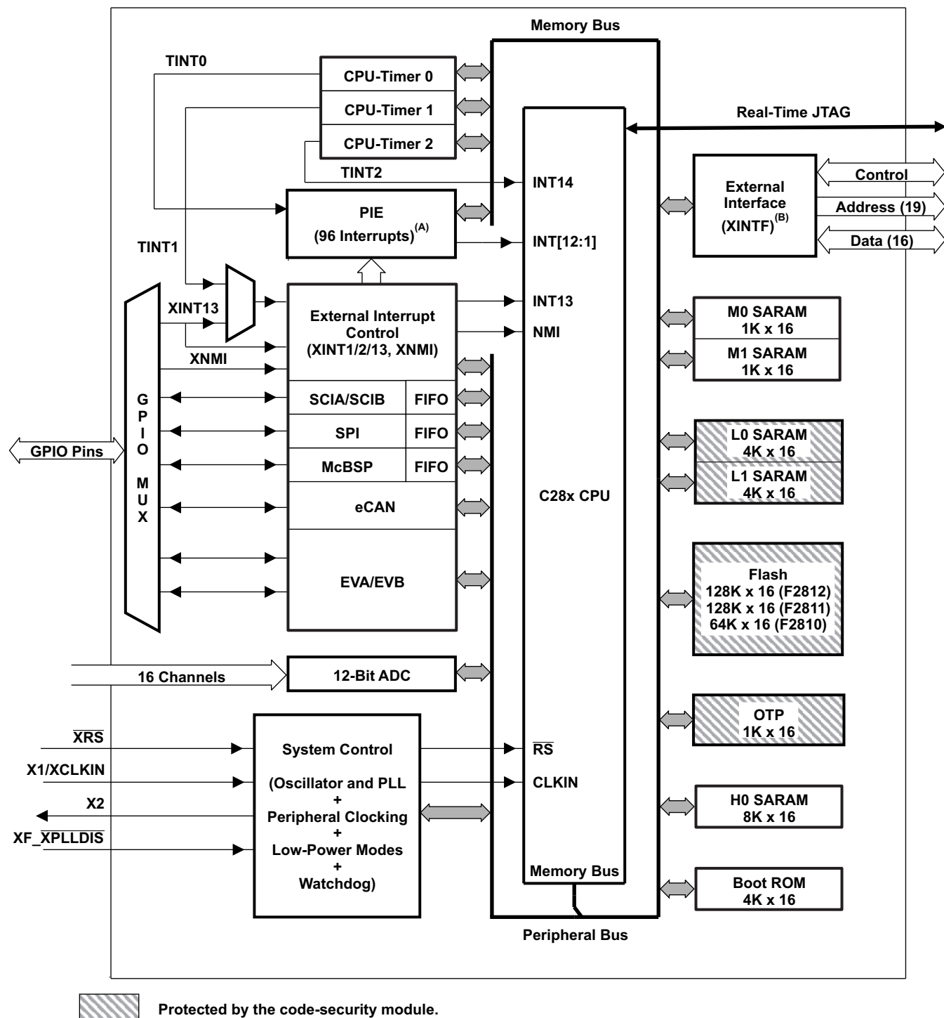
图 1-1. 功能方框图
