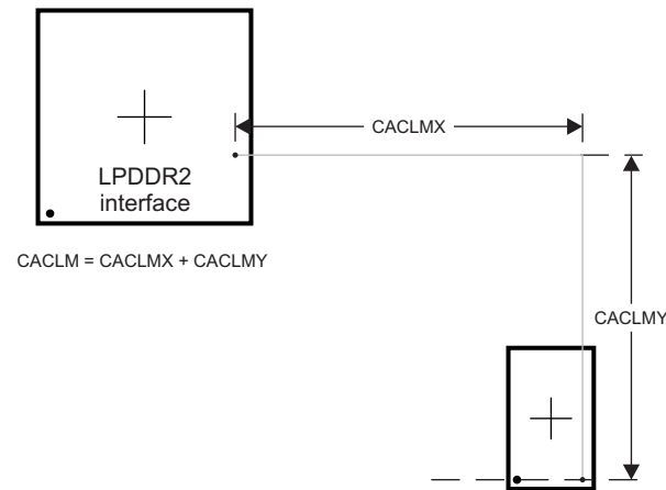
图 5-92. CACLM for LPDDR2 Interface
