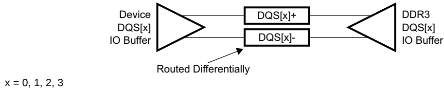
图 5-72. DQS[x] Topology
