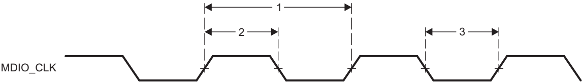
图 5-20. MDIO_CLK Timing
