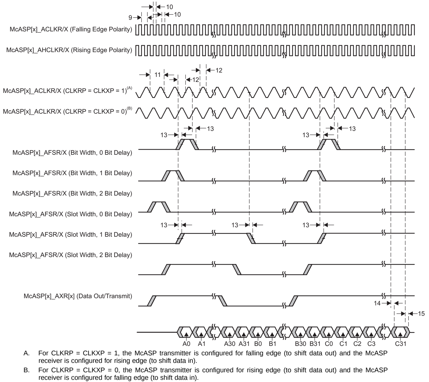
图 5-96. McASP Output Timing
