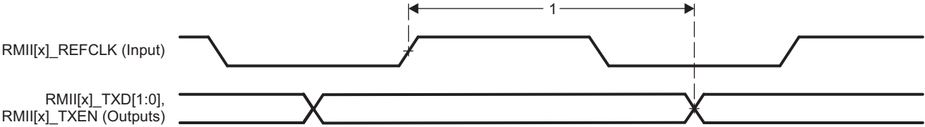
图 5-28. RMII[x]_TXD[1:0], RMII[x]_TXEN Timing - RMII Mode
