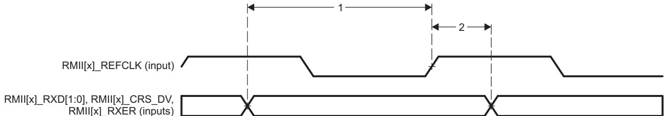
图 5-27. RMII[x]_RXD[1:0], RMII[x]_CRS_DV, RMII[x]_RXER Timing - RMII Mode
