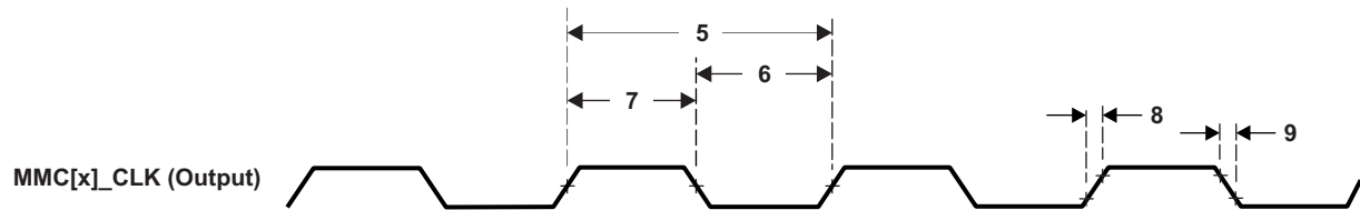
图 5-132. MMC[x]_CLK Timing
