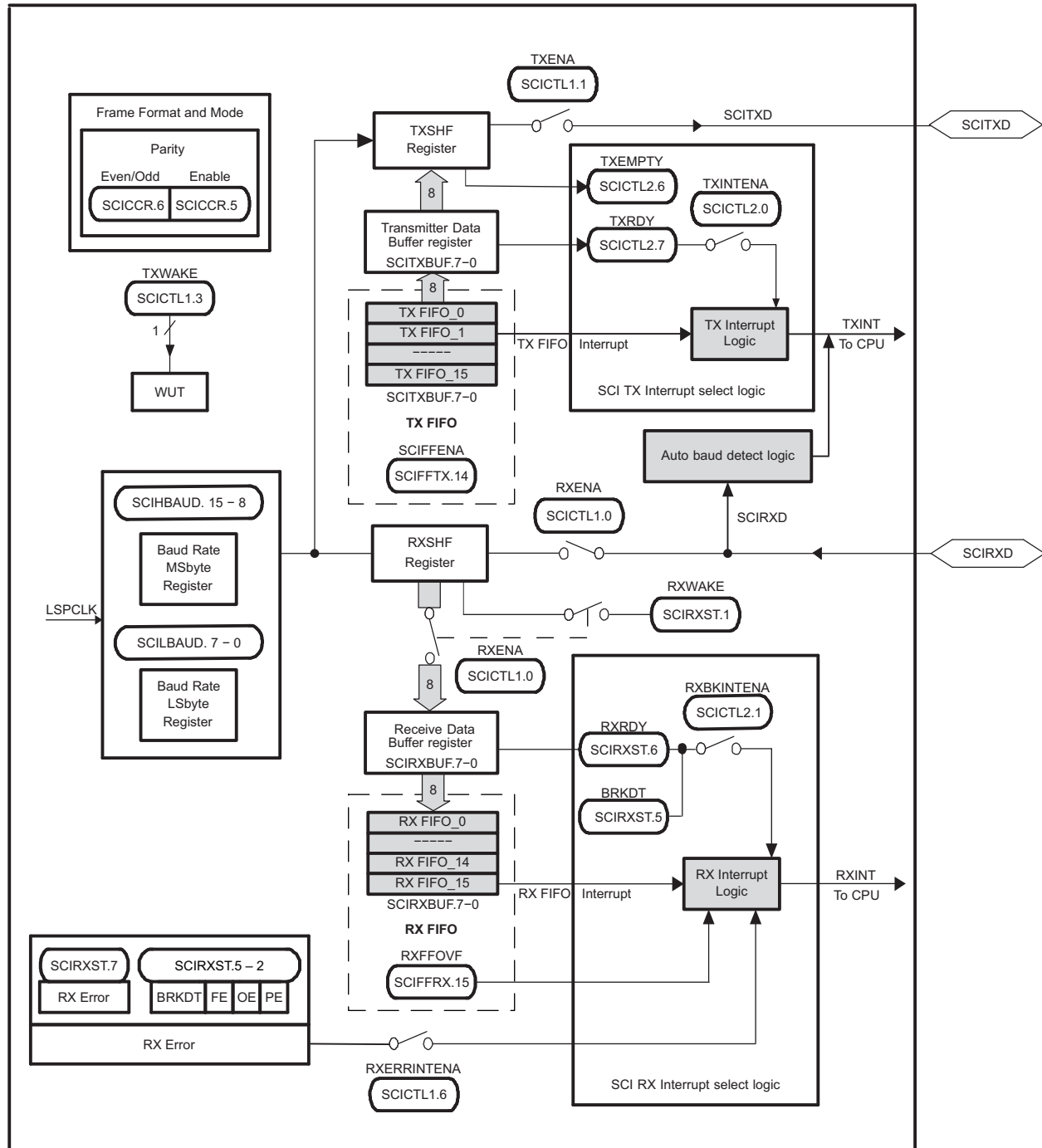
图 5-65. SCI Block Diagram
