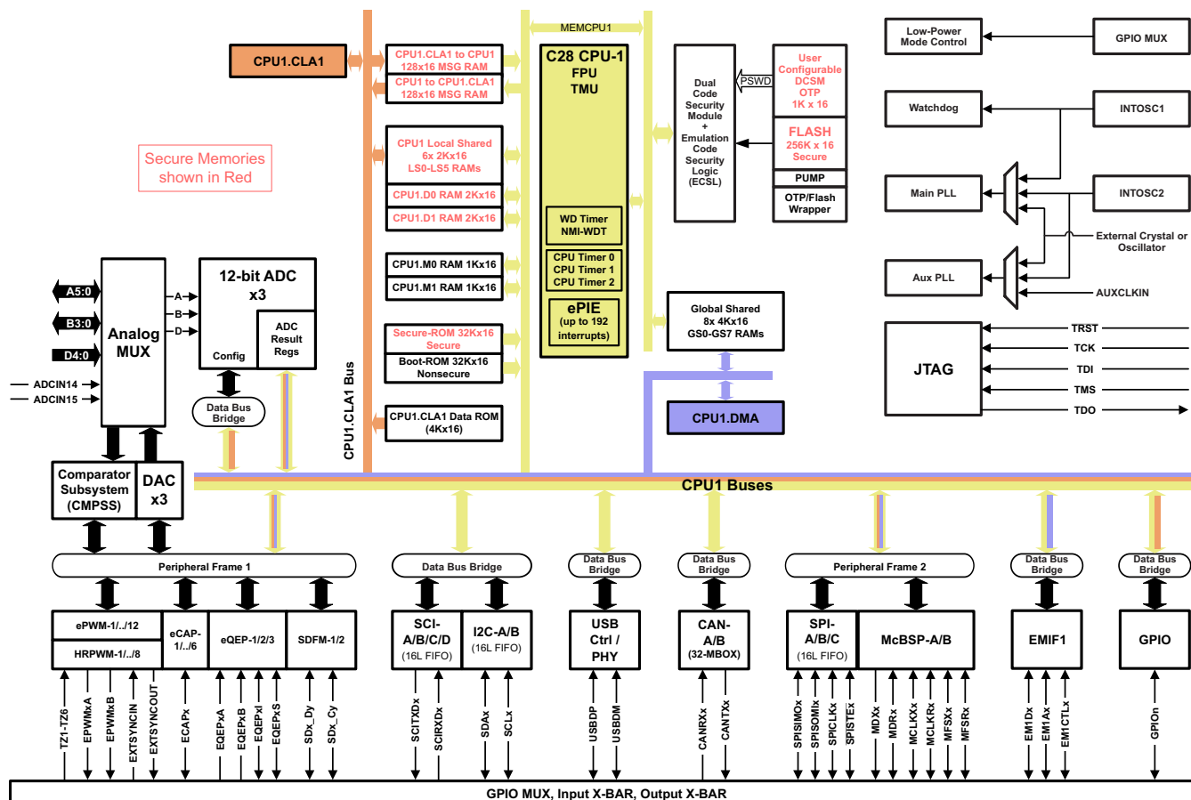
图 1-1. 功能方框图
