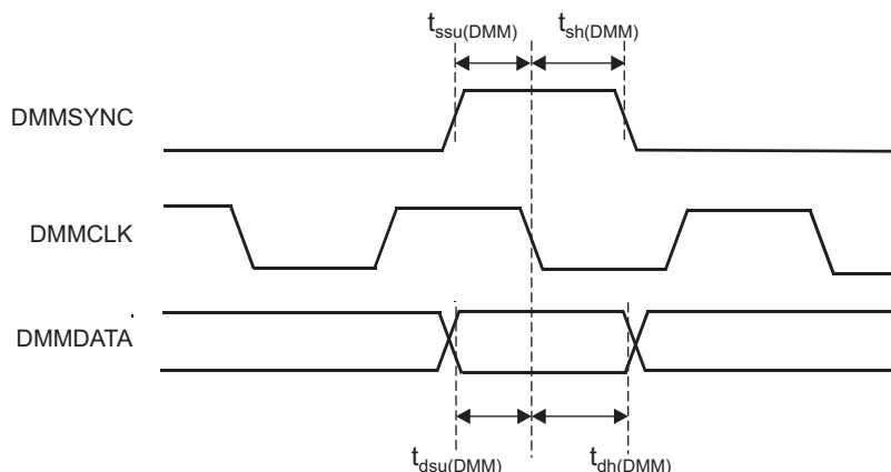
图 6-28. DMMDATA Timing
