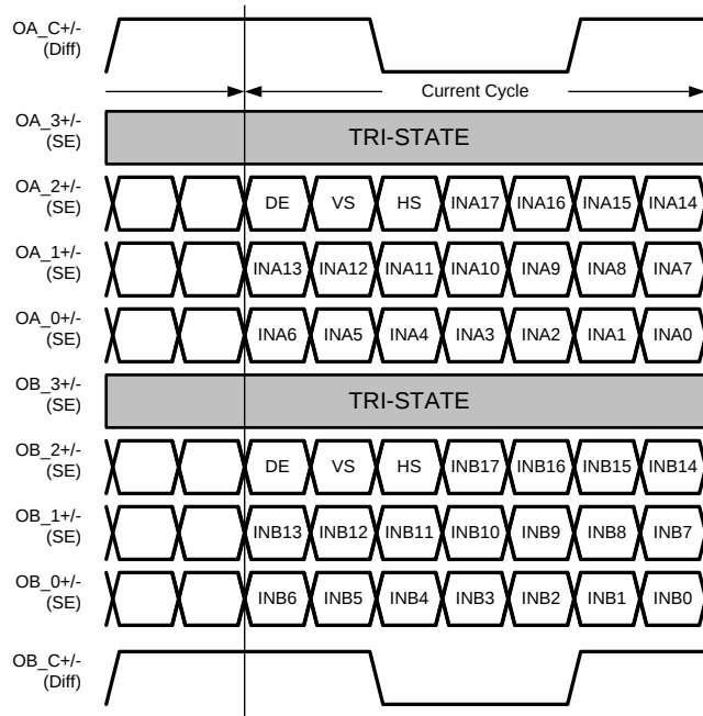
图 15. Dual Pixel / 18bpp LVDS Mapping
