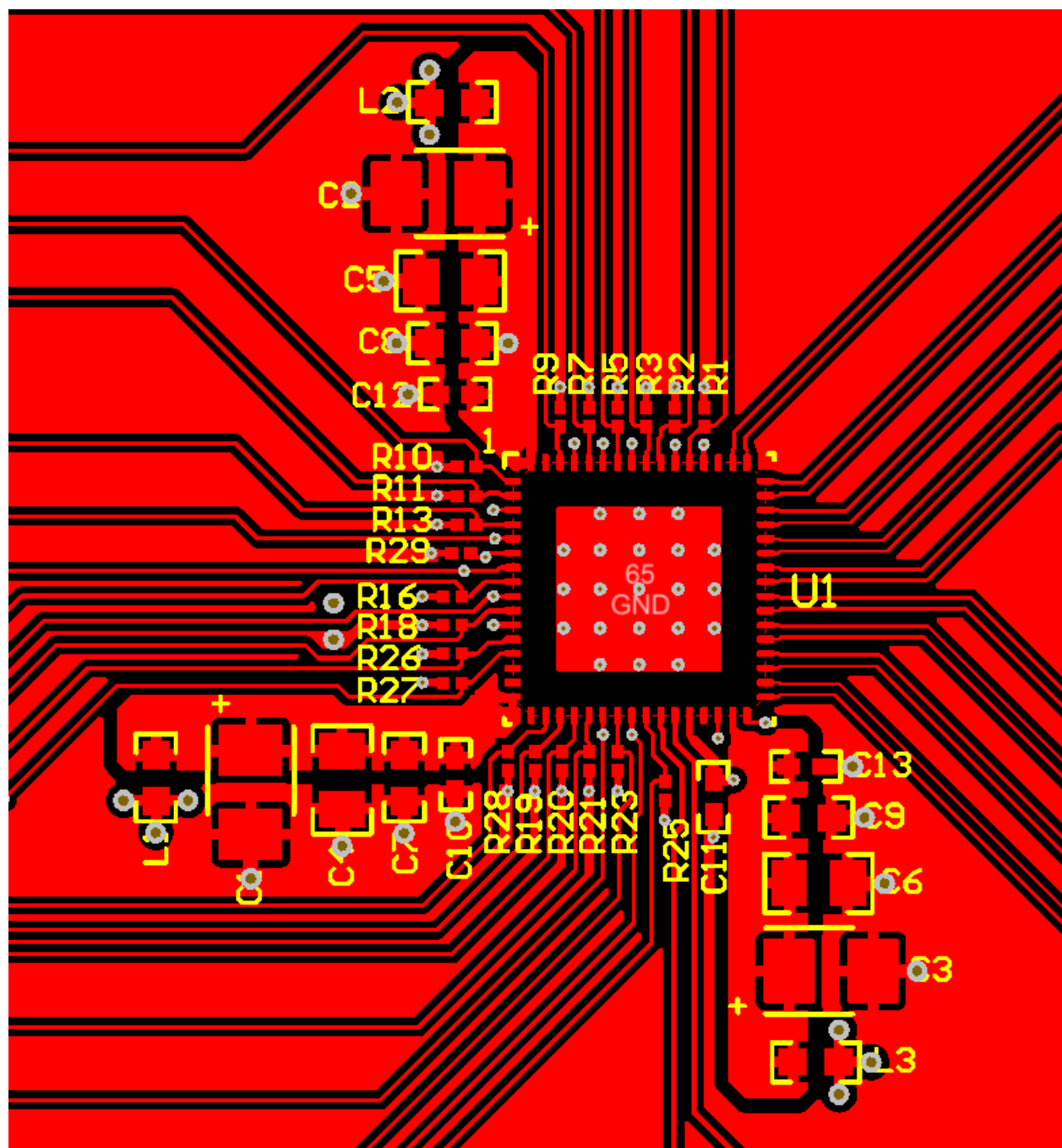
图 21. Layout Example
