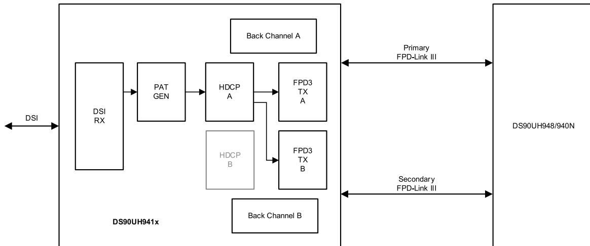
图 26. Dual-Link, 1:2 Mode
