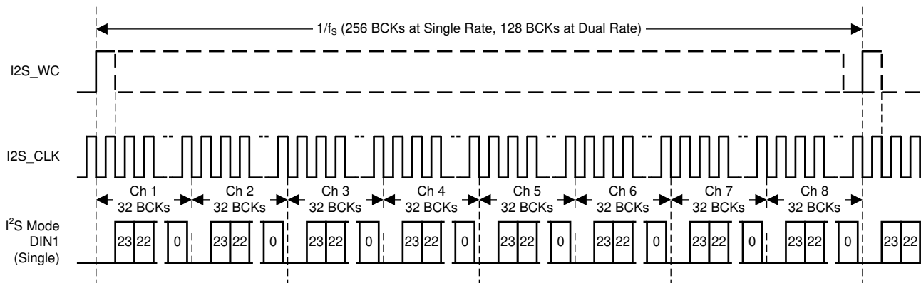
图 15. TDM Format
