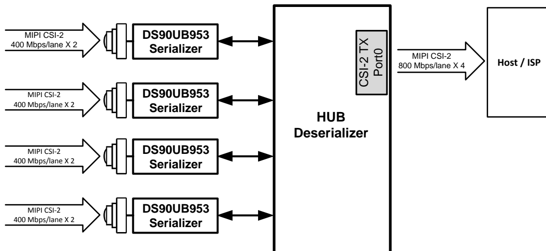
图 51. Four DS90UB953-Q1 Sensor Data Onto CSI-2 Over 1 Port
