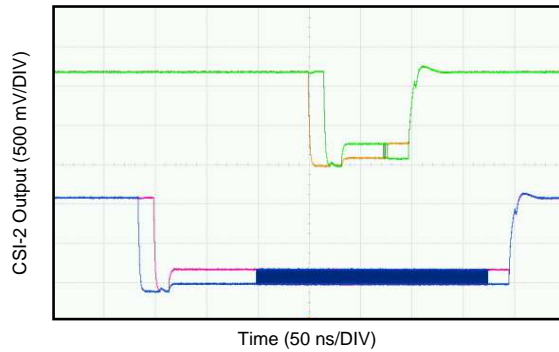
图 46. CSI-2 DATA and CLK Output
