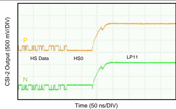
图 49. CSI-2 End of Transmission (EoT)
