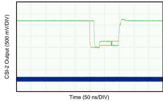
图 47. CSI-2 DATA and Continuous CLK Output
