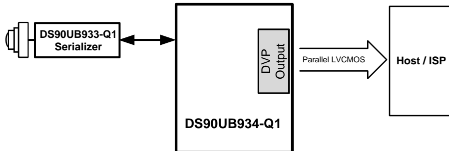
图 30. DS90UB933-Q1 Camera Data to 1 Rx Port
