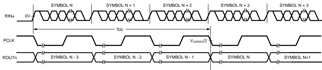
图 6. Deserializer Delay
