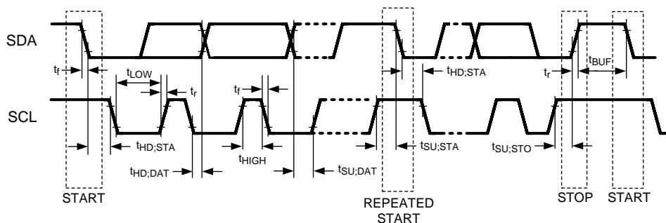
图 21. Basic Operation
