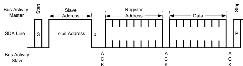
图 20. Serial Control Bus — WRITE
