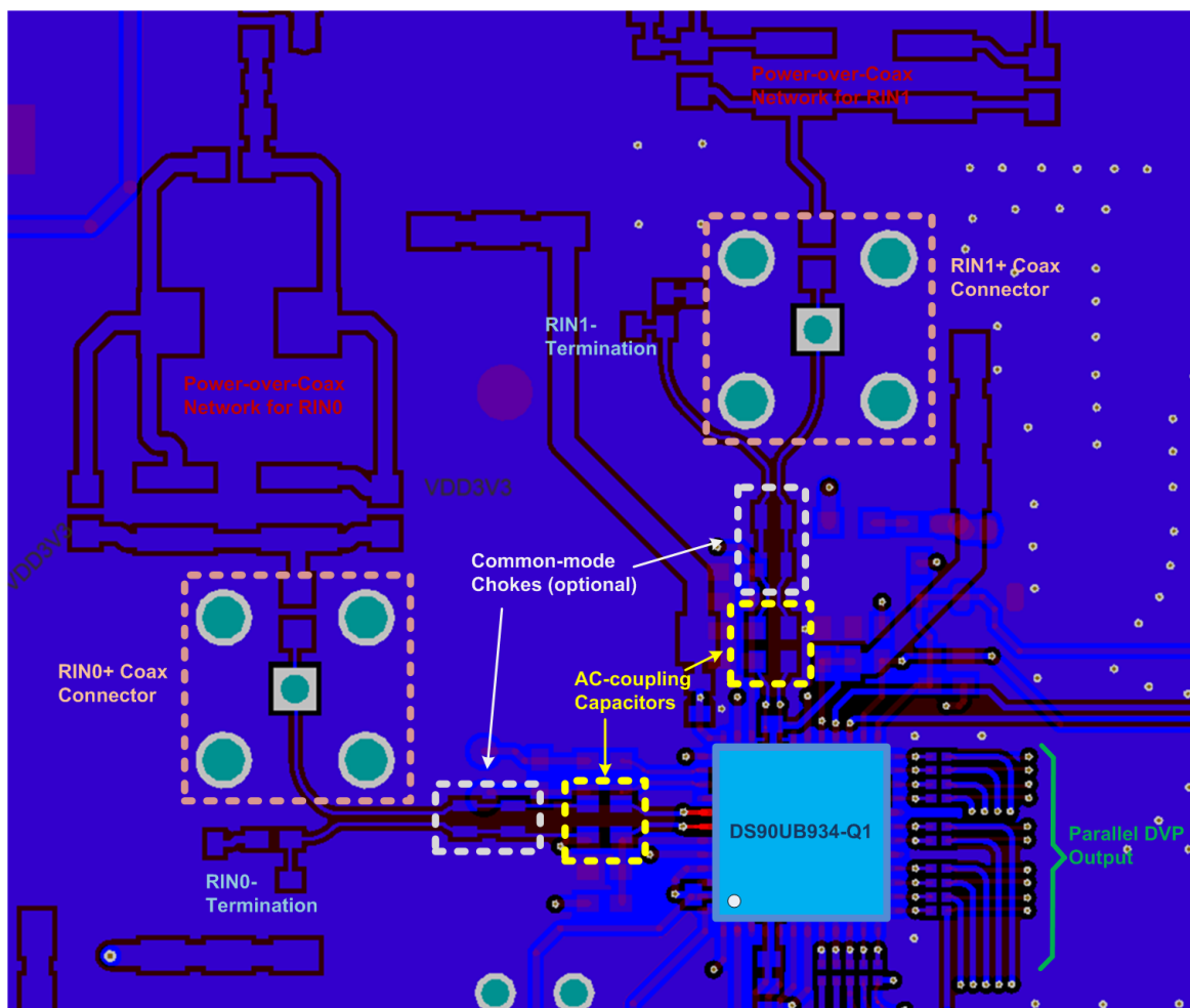
图 33. DS90UB934-Q1 Example PCB Layout
