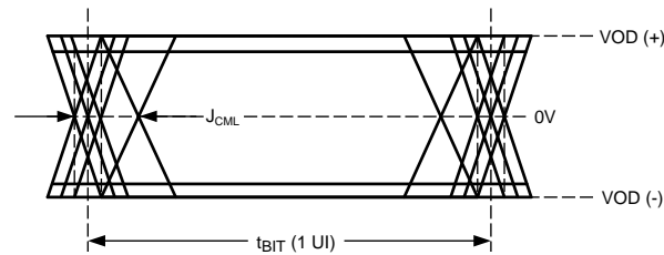
图 15. CMLOUT Output Driver
