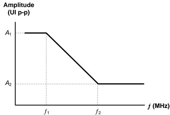
图 14. Input Jitter Tolerance Plot
