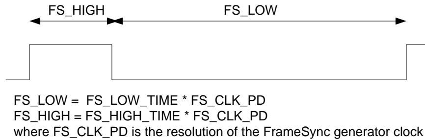
图 16. Internal FrameSync Signal
