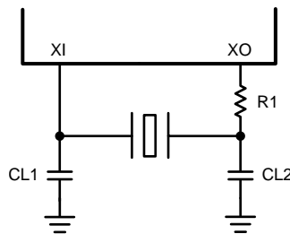
图 28. Crystal Oscillator Circuit
