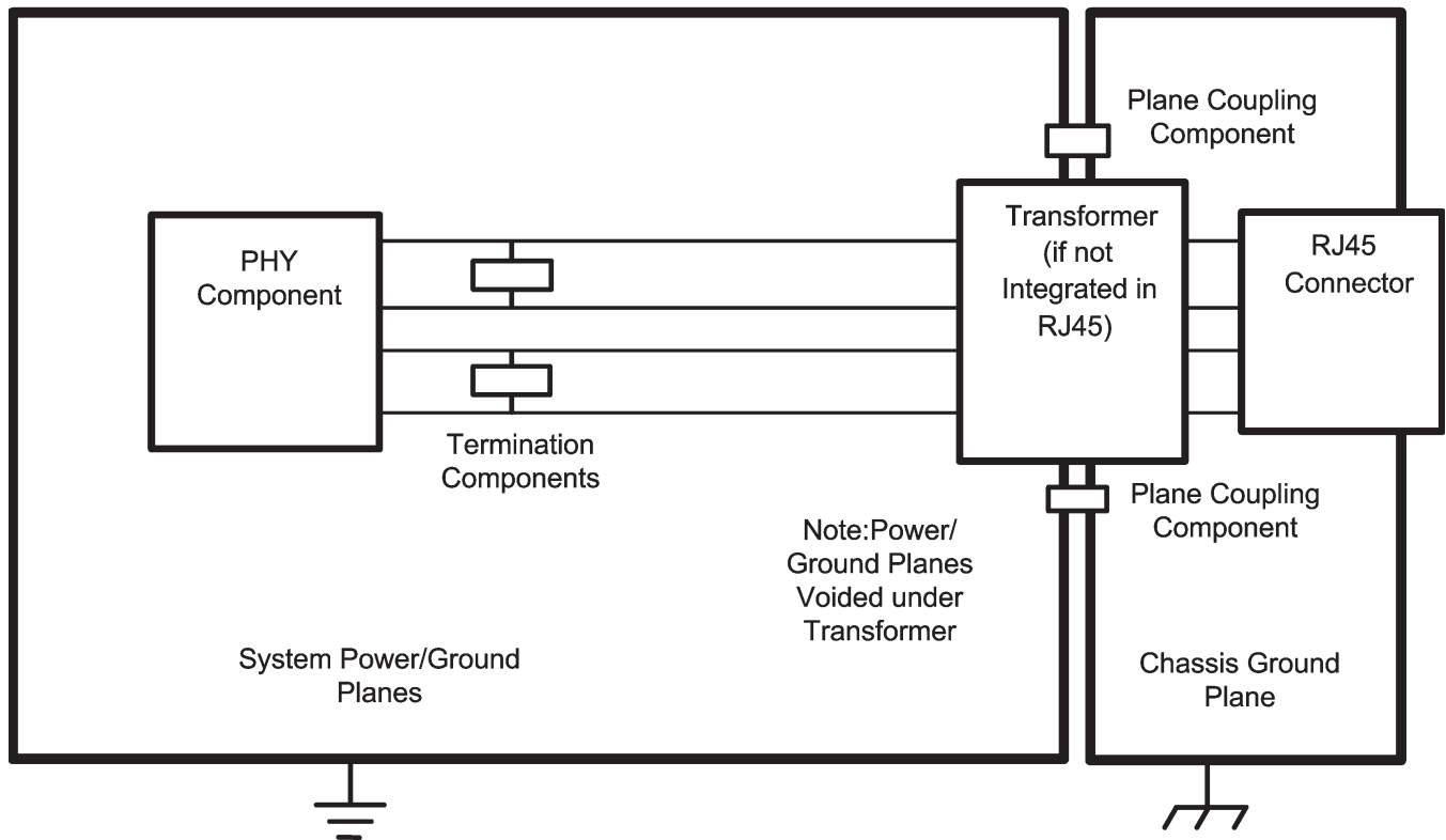
图 8-5. Layout Example
