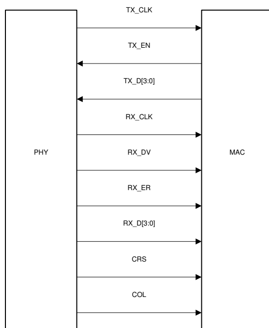
图 19. MII Signaling
