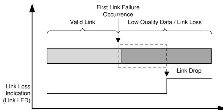
图 23. Fast Link-Drop
