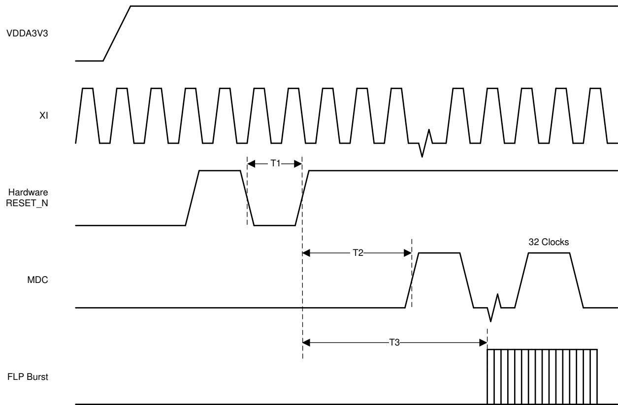
图 2. Reset Timing (POR)
