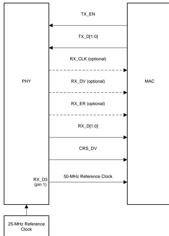
图 26. RMII Master Signaling
