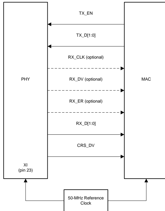
图 25. RMII Slave Signaling
