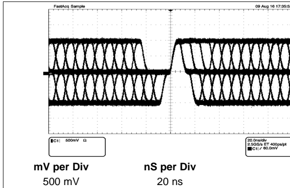
图 17. 100BASE-TX PMD Eye Waveform
