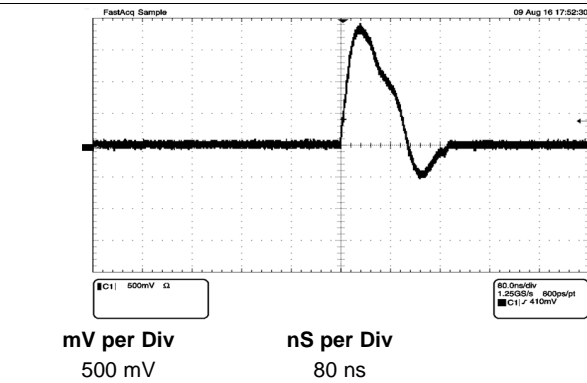
图 18. 10BASE-Tc Link Pulse Waveform
