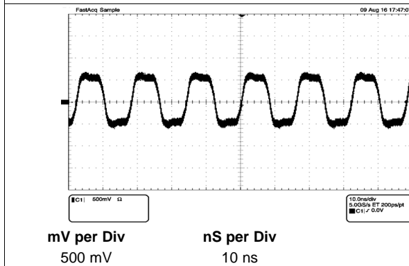
图 19. 100BASE-FX Waveform
