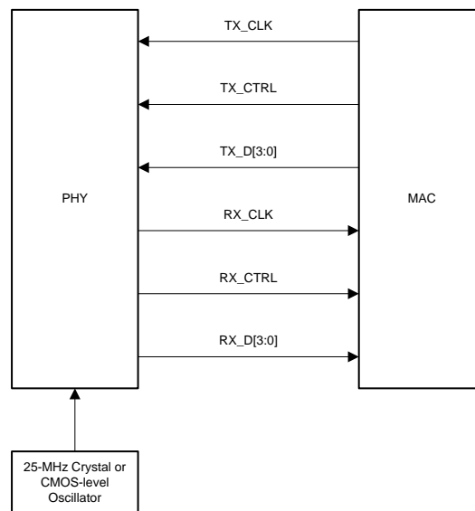
图 27. RGMII Signaling
