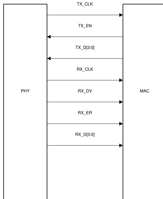
图 7-2. MII Signaling
