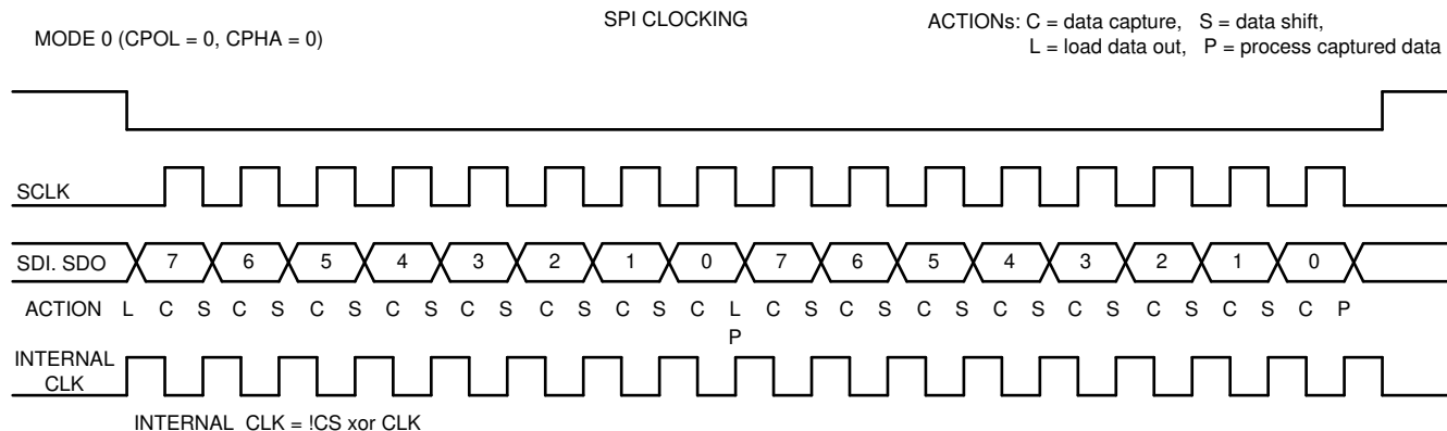
图 33. SPI Clocking
