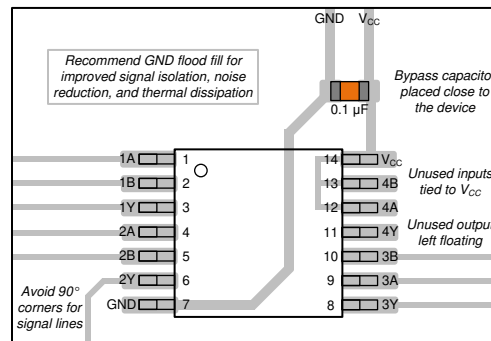
图 11. Example layout for the SN74HCS08-Q1
