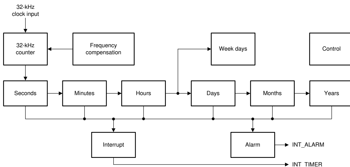
图 5-20. RTC Block Diagram
