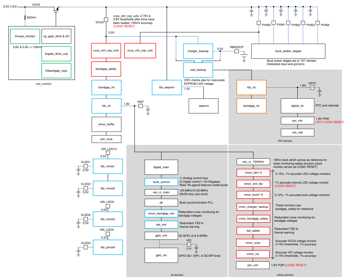
图 1-2. 内部电源树图
