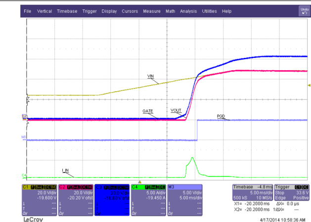
图 31. Start-Up
