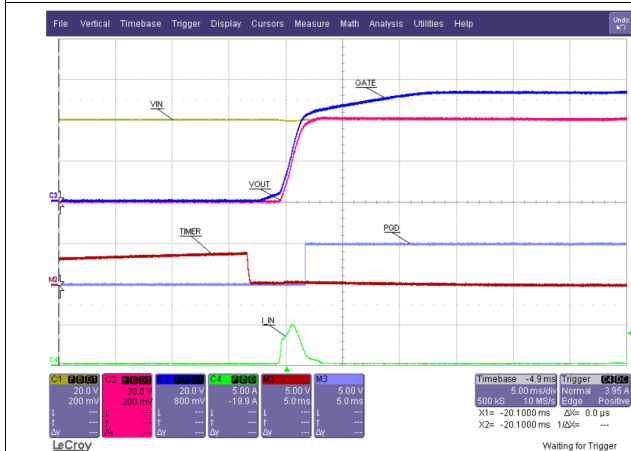
图 28. Insertion Delay
