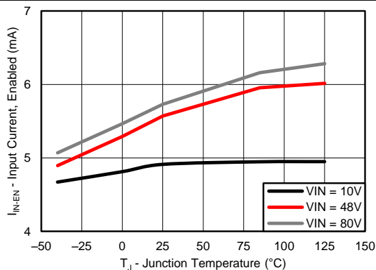
图 2. Input Current vs VIN and T_J
