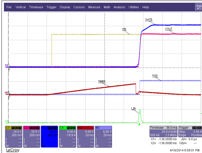
图 28. Insertion Delay
