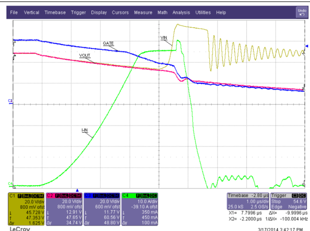
图 48. Loadstep
