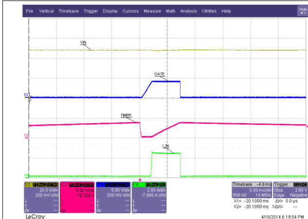
图 30. Start-Up
