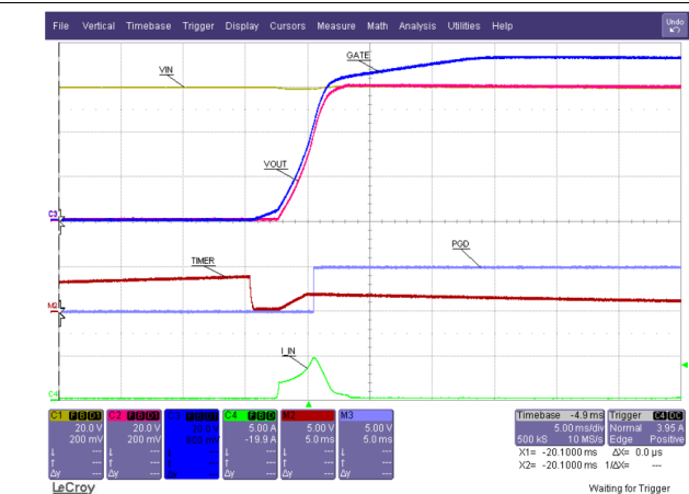
图 29. Start-Up
