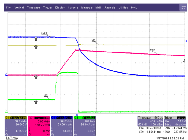
图 48. Loadstep
