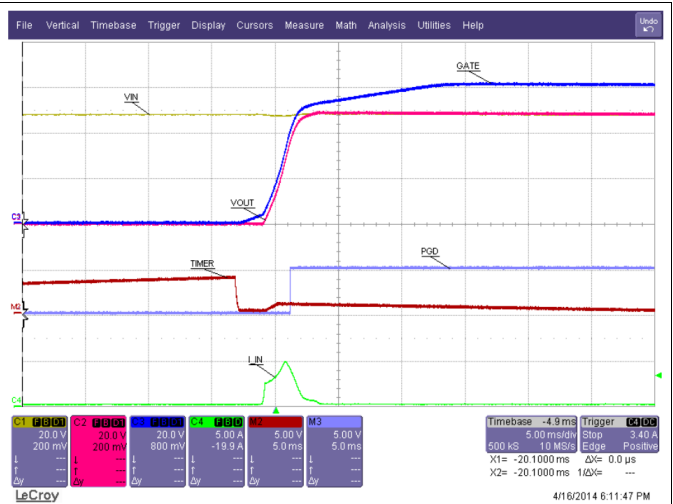
图 29. Start-Up
